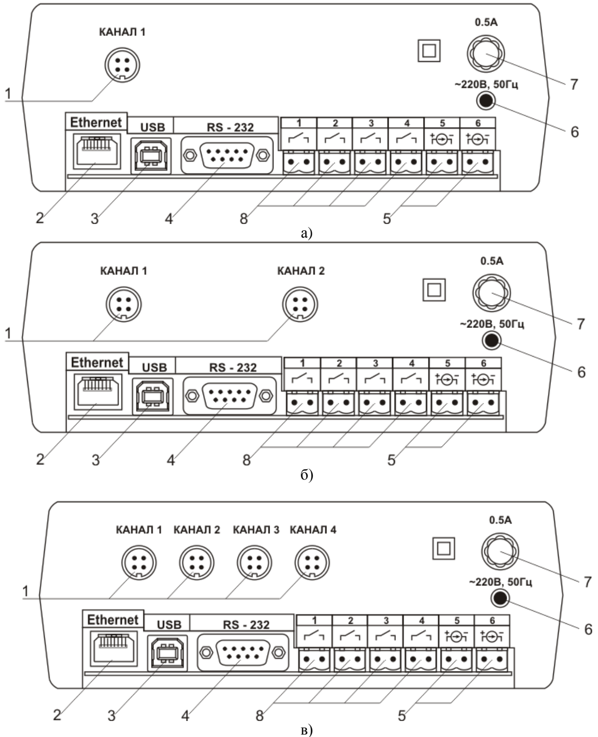
Рисунок 3.4 Вид задних панелей газоанализаторов ПКГ-4 /X-T-K-4P-2A-E (3):
