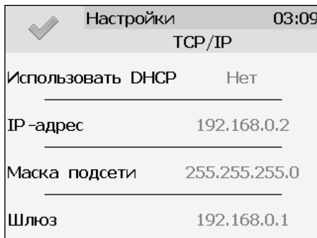
Рисунок 6.24 Экран настройки TCP/IP
