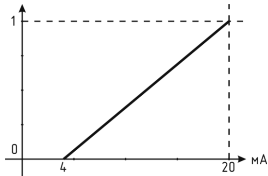
Рисунок 3.15 Линейный выход 4...20 мА с диапазоном 0...1%
