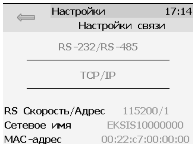
Рисунок 6.23 Экран настроек связи (ПКГ-4 /Х-Т-К-4Р-2А-Е)
