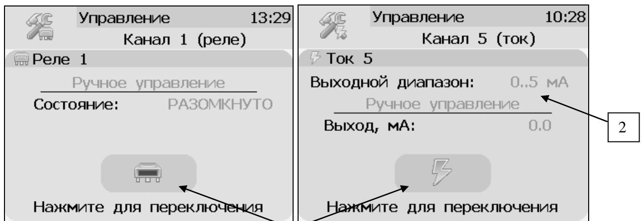
Рисунок 6.11 Виды экрана первого и пятого канала управления
