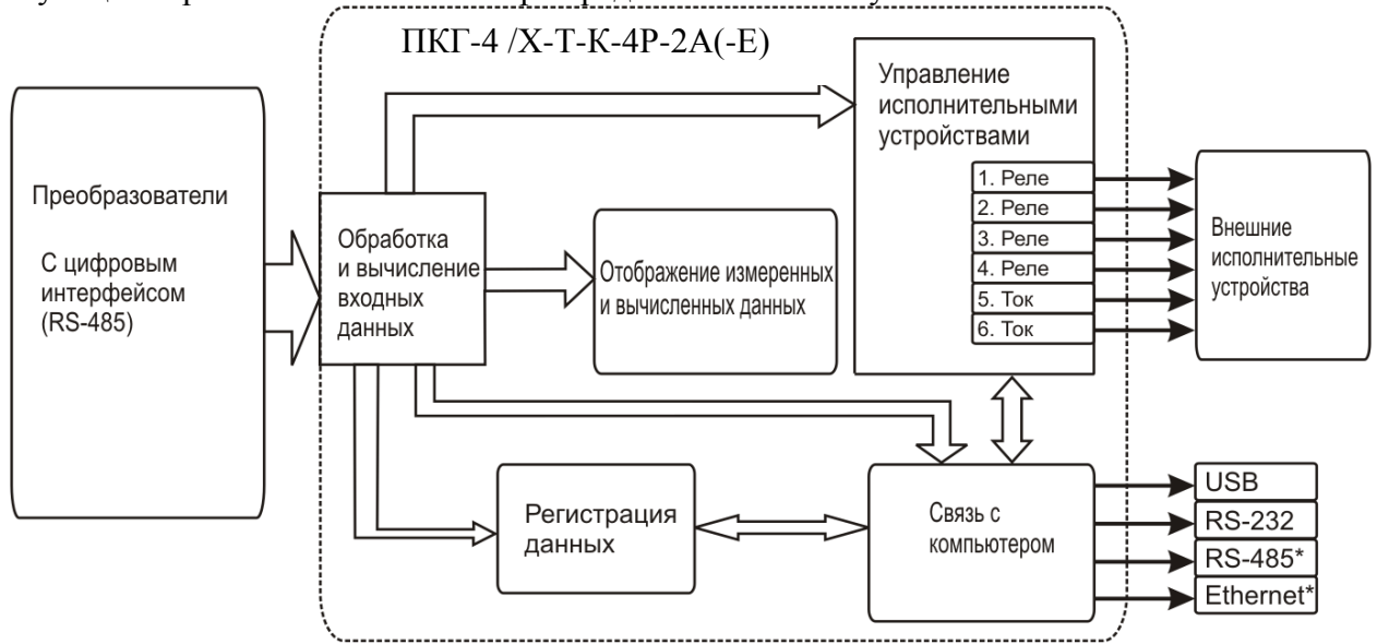
Рисунок 3.11 Функционирование газоанализатора
