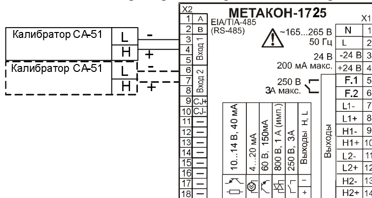
Рисунок А.7 – Схема подключения приборов для проведения поверки по сигналам тока
