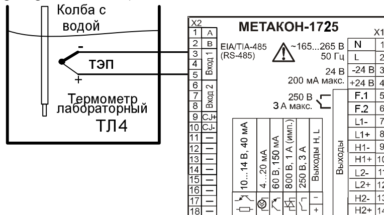
Рисунок А.10 – Схема подключения прибора для определения основной погрешности компенсации влияния температуры холодных спаев
