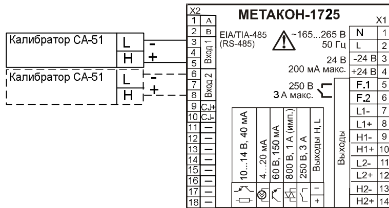
Рисунок А.6 – Схема подключения приборов для проведения поверки по сигналам напряжения
