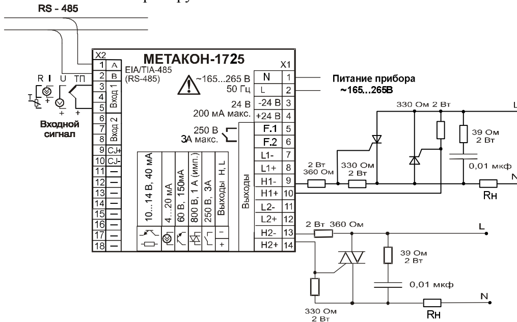
Рисунок 13 – Электрическая схема подключения внешнего симистора и тиристоров к прибору МЕТАКОН-1725-2С/2Р-У-1
