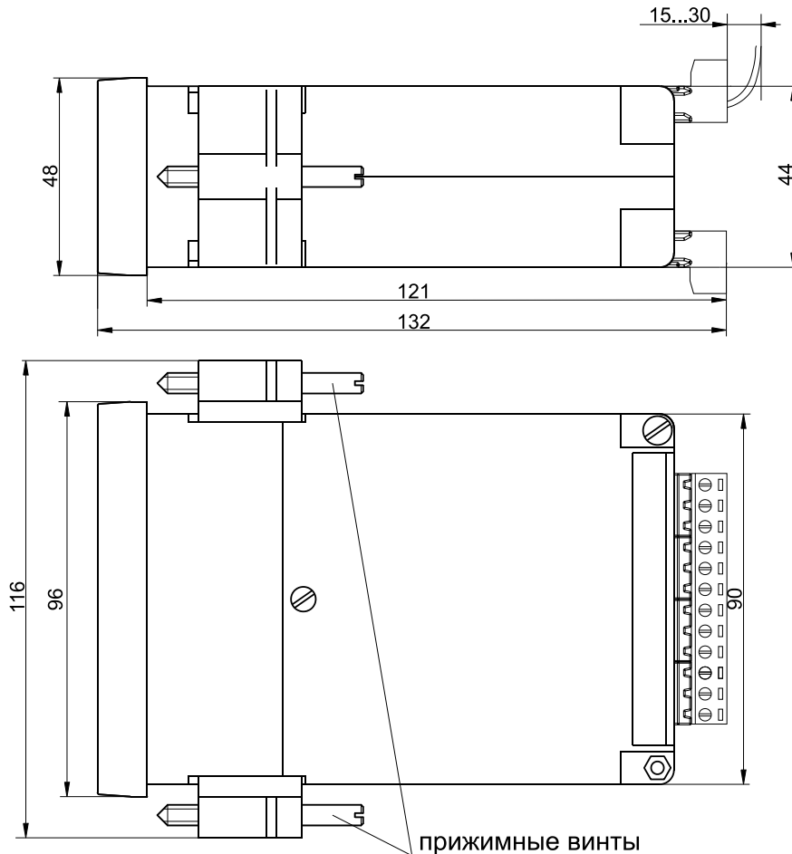
Рисунок 9 – Габаритные размеры измерителя-регулятора МЕТАКОН-17Х5
