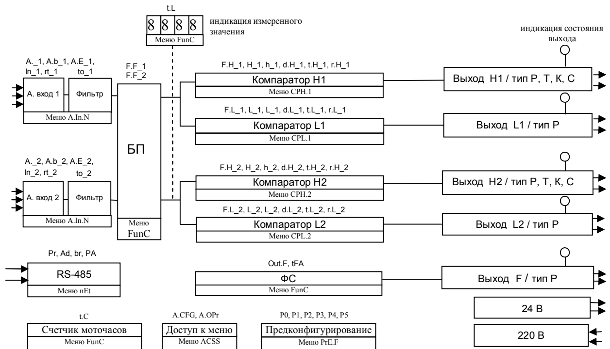
Рисунок 2 – Функциональная структура приборов М-1725-2P/2P, 2T/2P, 2K/2P, 2C/2P
