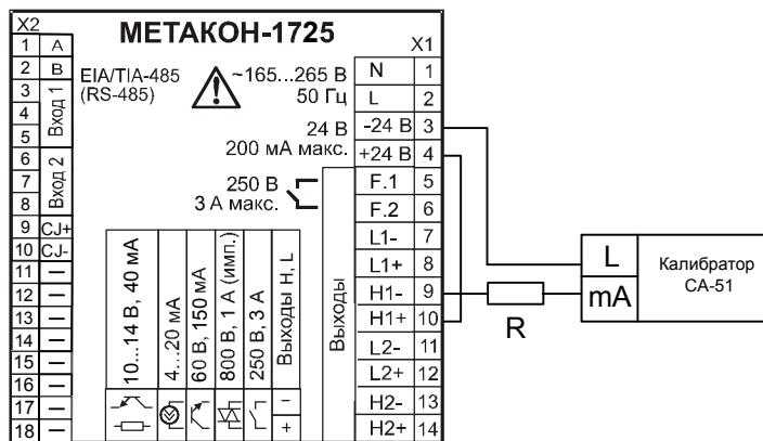
Рисунок А.9 – Схема подключения прибора для поверки основной погрешности установления тока в токовом выходе, где R – резистор С2-33Н-0,125-200 Ом \pm 5 %.
