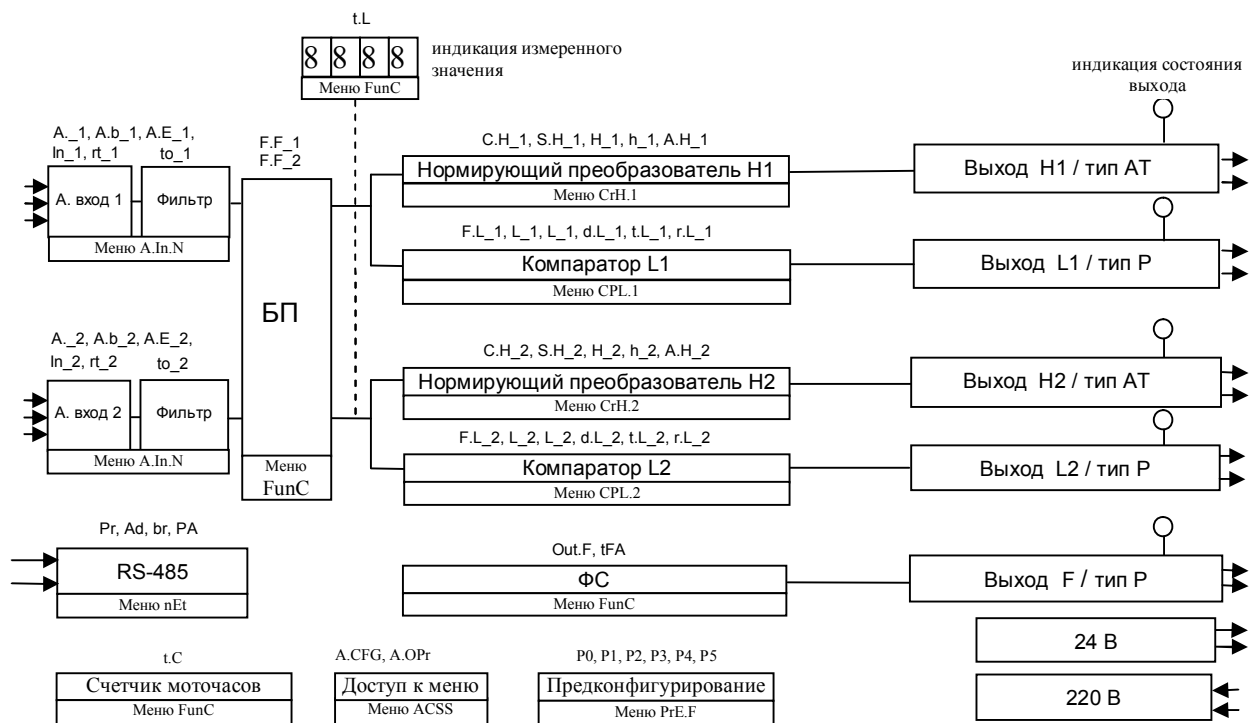
Рисунок 3 – Функциональная структура прибора М-1725-2АТ/2P
