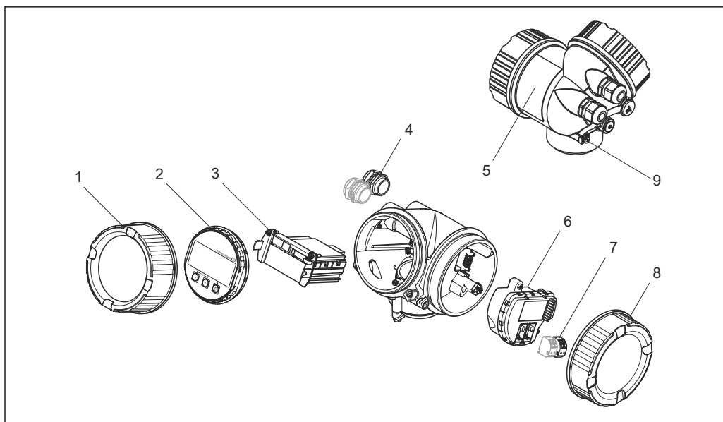
2 Конструкция корпуса электроники
