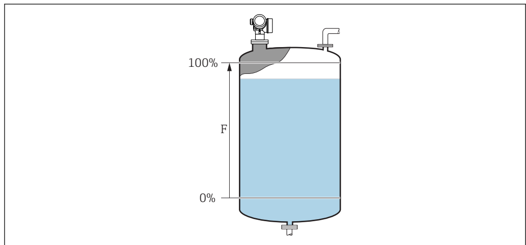
23 Калибровка полной емкости (F) для измерения уровня в жидкостях
