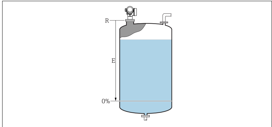
22 Калибровка пустой емкости (E) для измерения уровня в жидкостях
