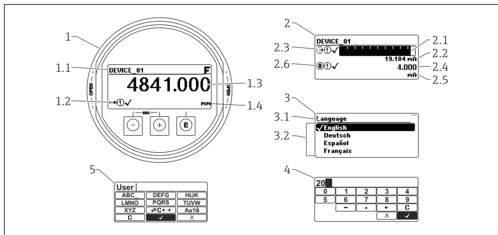
16 Внешний вид дисплейного и рабочего модуля при работе в локальном режиме
