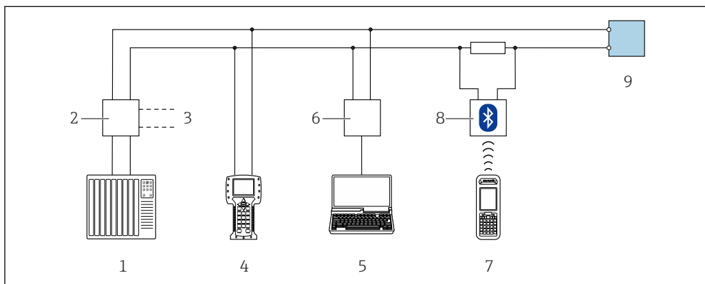
15 Варианты дистанционного управления по протоколу HART
