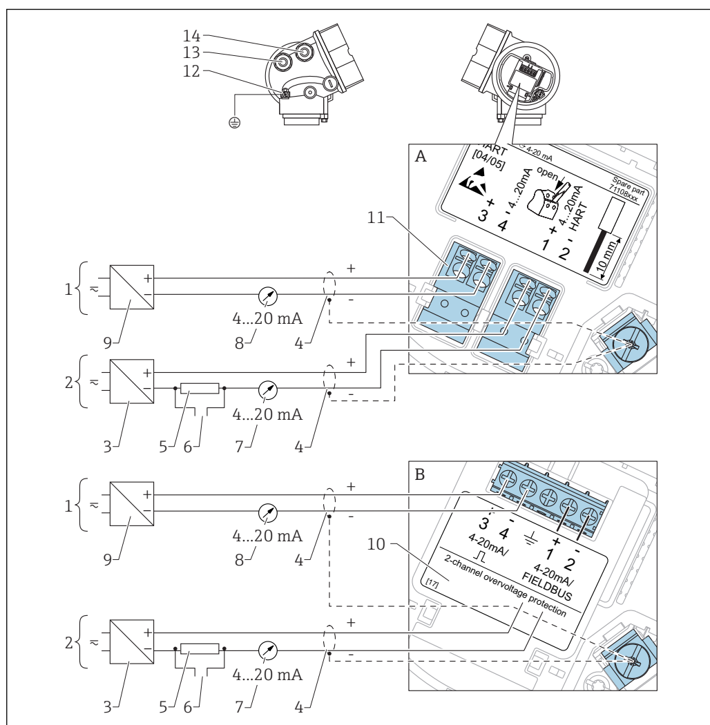
7 Назначение клемм: 2-проводная, 4...20 мА HART, 4...20 мА
