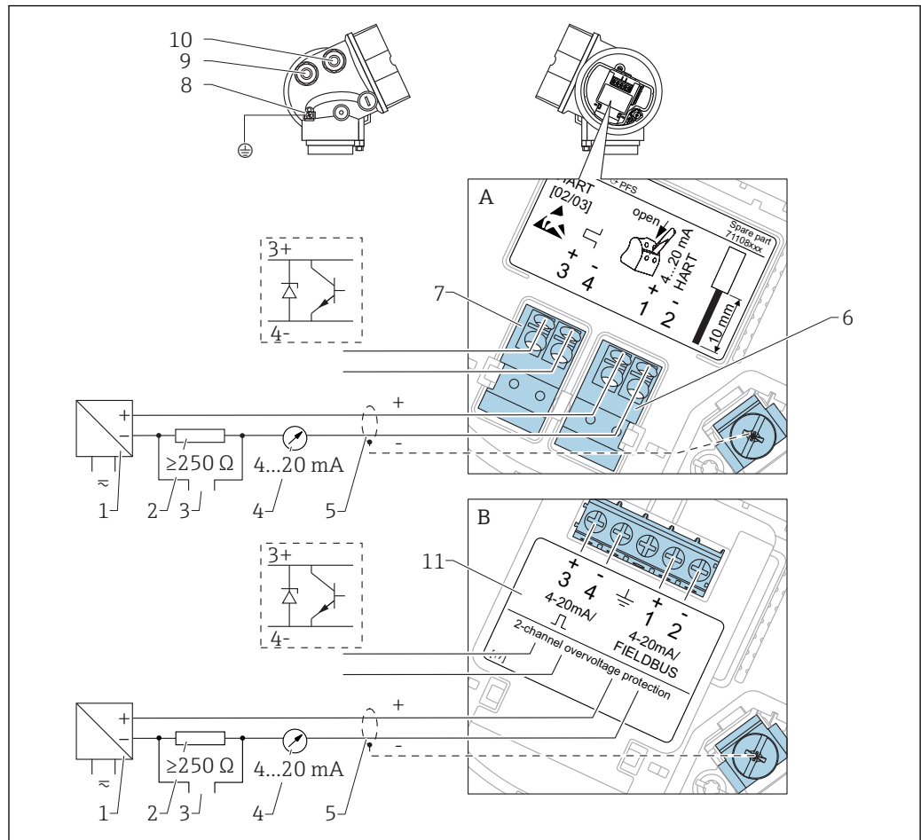
6 Назначение 2-проводной клеммы: 4–20 мА HART, переключающий выход
