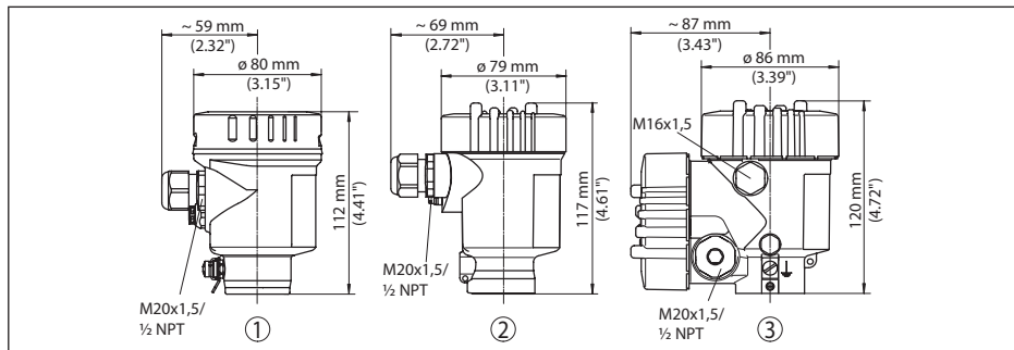
Рис. 44: Корпуса в исполнении IP 66/IP 68 (0,2 bar) - с установленным модулем индикации и настройки корпус выше на 9 мм/0.35 in
