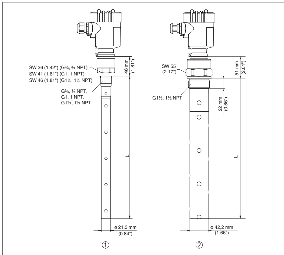
Рис. 46: VEGAFLEX 81, резьбовое исполнение
