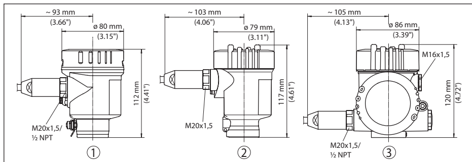
Рис. 45: Корпуса в исполнении IP 66/IP 68 (1 bar) - с установленным модулем индикации и настройки корпус выше на 9 мм/0.35 in
