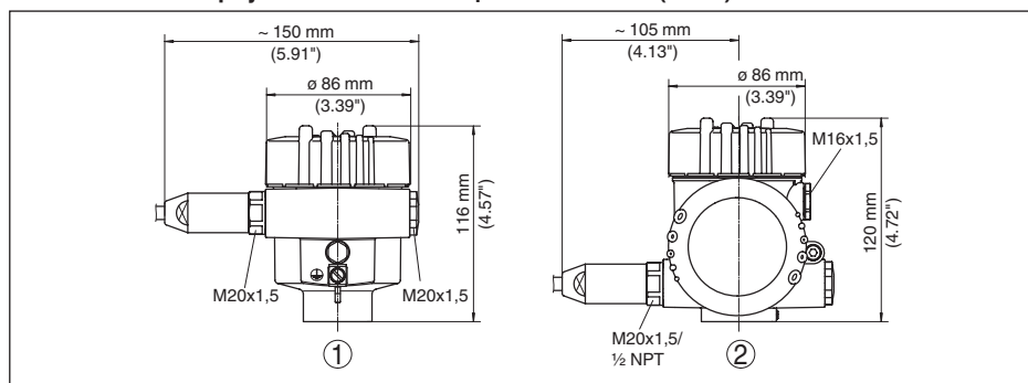
Рис. 43: Корпуса в исполнении IP 66/IP 68 (1 bar) - с установленным модулем индикации и настройки корпус выше на 9 mm/0.35 in
