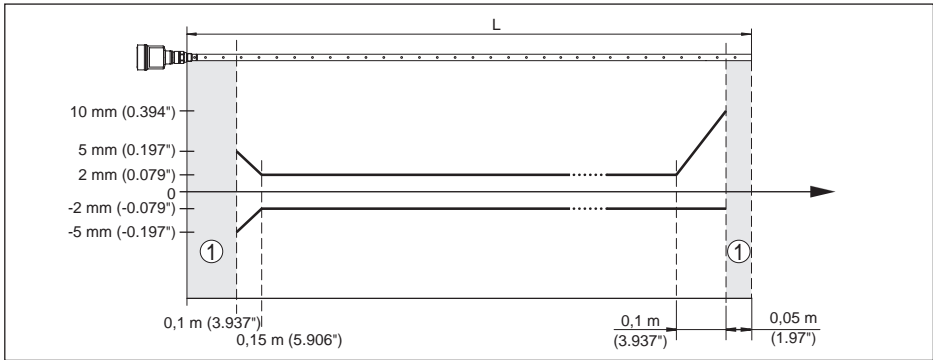
Рис. 38: Погрешность измерения VEGAFLEX 81 в коаксиальном исполнении (среда - масло)
