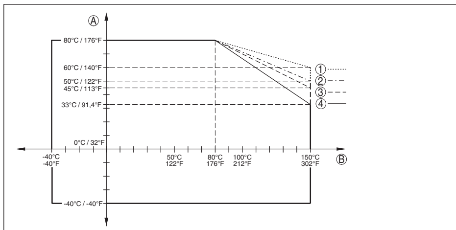
Рис. 39: Температура окружающей среды - температура процесса, стандартное исполнение
