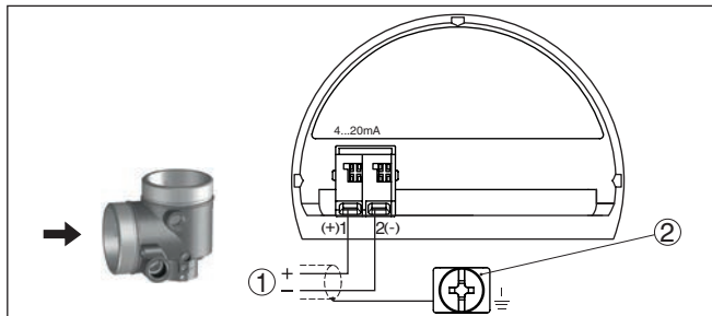
Рис. 13: Отсек подключения (двухкамерный корпус, исполнение с комбинированной взрывозащитой Ex d ia)
