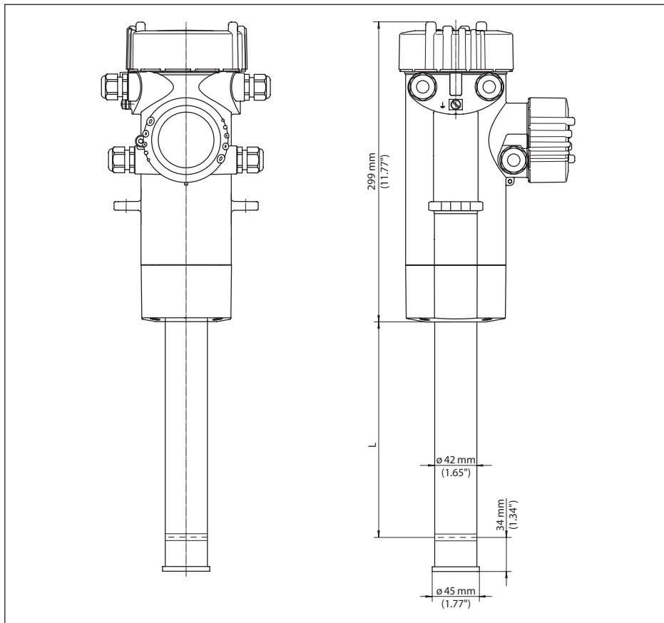
Рис. 32: FIBERTRAC 31
