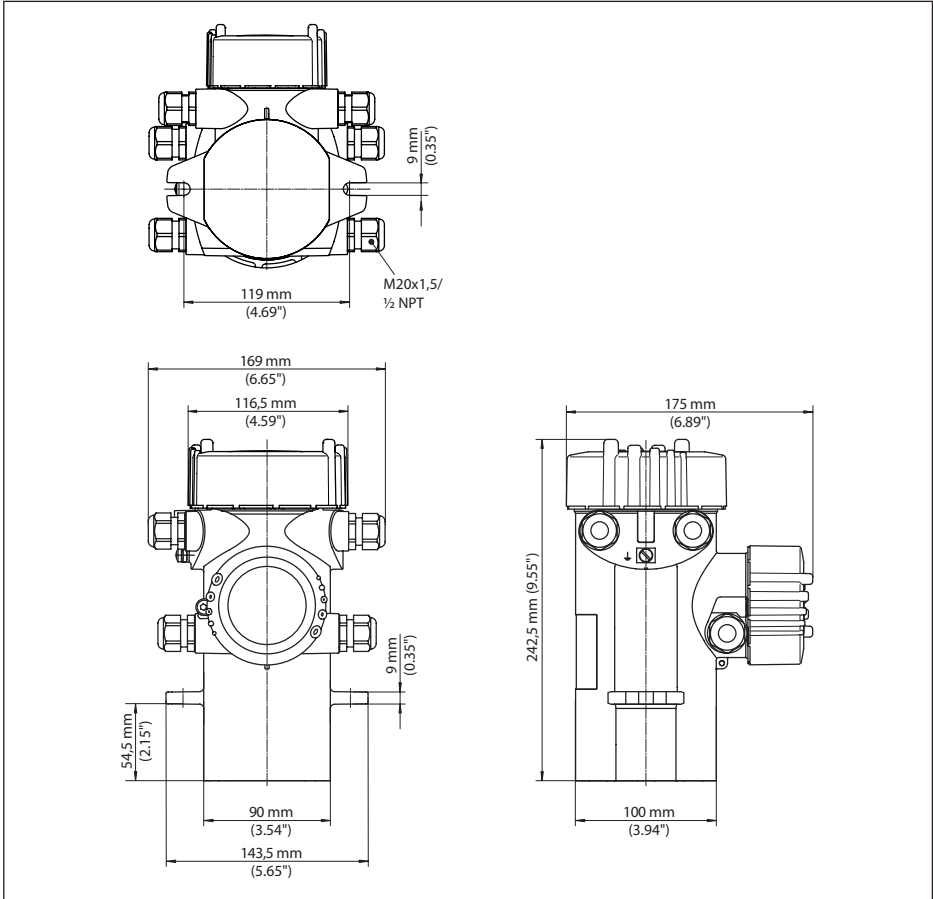
Рис. 31: Корпус из алюминия или нержавеющей стали (точное литье)
