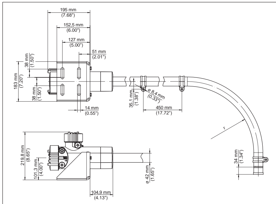
Рис. 33: FIBERTRAC 31 с поставляемыми в комплекте монтажными принадлежностями
