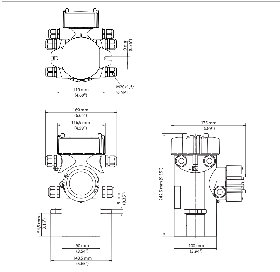
Рис. 21: Корпус из алюминия или нержавеющей стали (точное литье)
