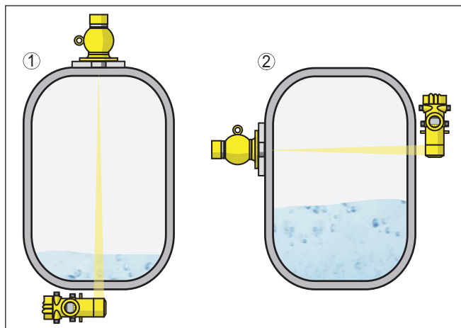
Рис. 2: Возможности применения MINITRAC 31
