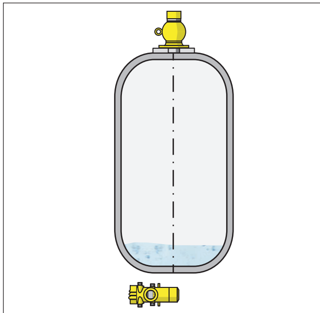
Рис. 5: Измерение уровня - обнаружение остатков в резервуаре-хранилище
