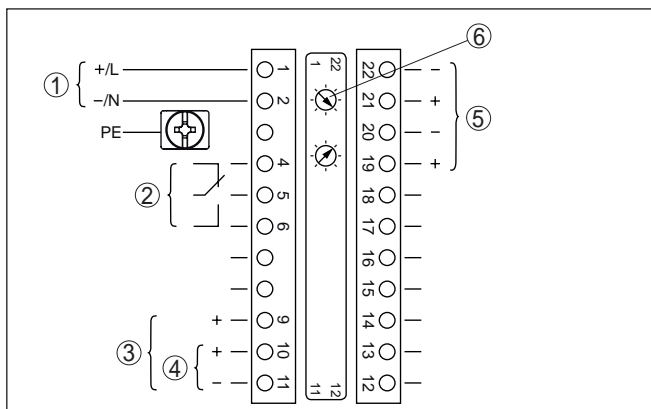
Рис. 11: Отсек электроники и подключения у устройств без взрывозащиты и устройств с не искробезопасным токовым выходом
