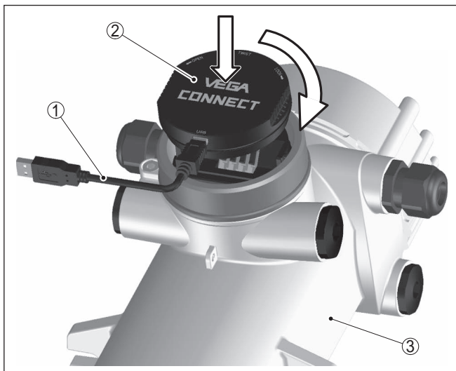
Рис. 17: Подключение ПК через интерфейсный адаптер прямо к датчику
