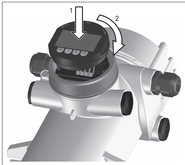
Рис. 15: Установка модуля индикации и настройки
