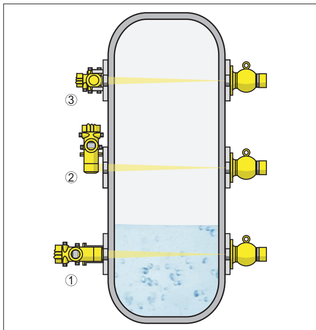
Рис. 4: Монтажная позиция - сигнализация предельного уровня
