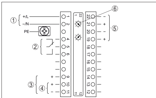
Рис. 7: Отсек электроники и подключения у устройств без взрывозащиты и устройств с не искробезопасным токовым выходом
