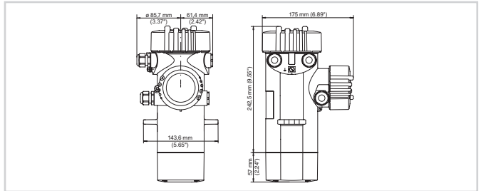
Размеры MINITRAC 31
