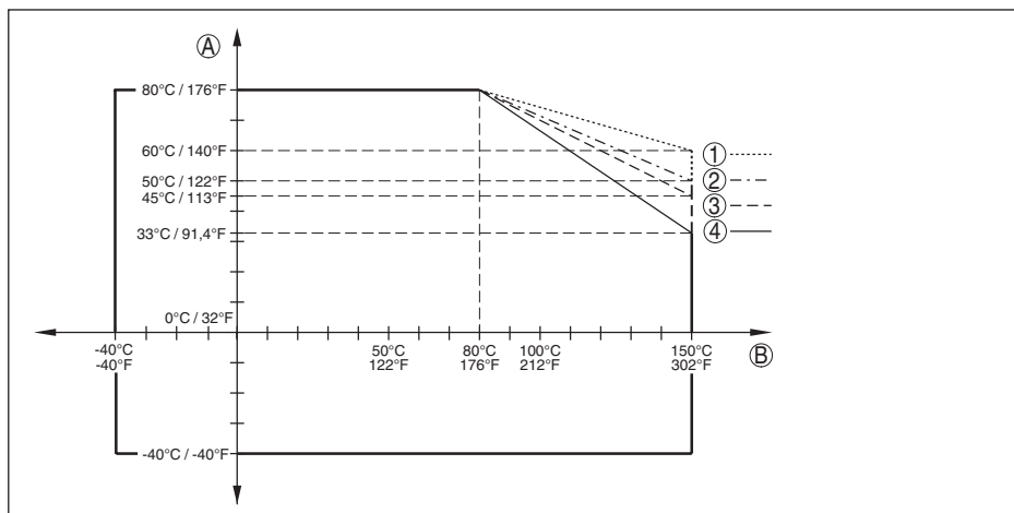
Рис. 36: Температура окружающей среды - температура процесса, стандартное исполнение
