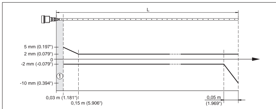
Рис. 34: Погрешность измерения VEGAFLEX 81 в коаксиальном исполнении (среда - вода)
