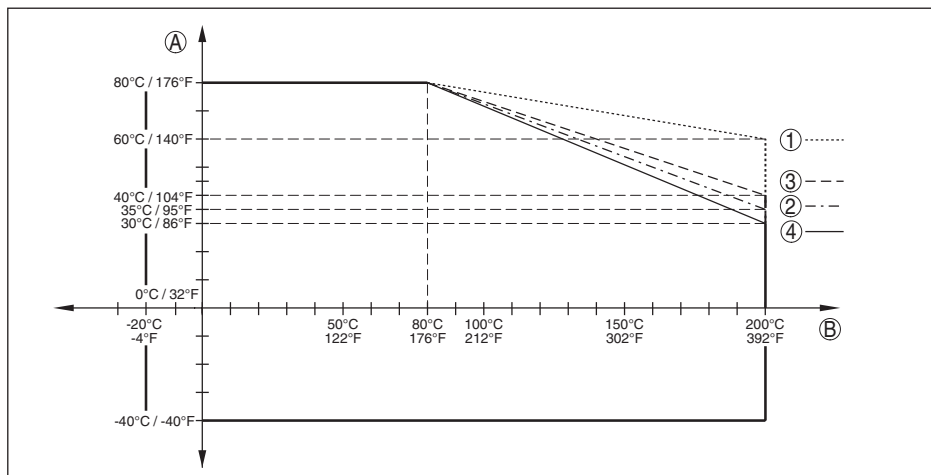
Рис. 37: Температура окружающей среды - температура процесса, исполнение с температурной вставкой
