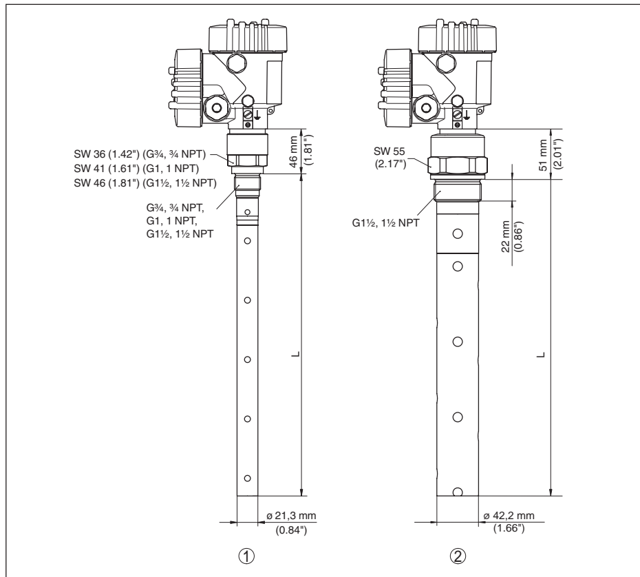
Рис. 39: VEGAFLEX 81, резьбовое исполнение
