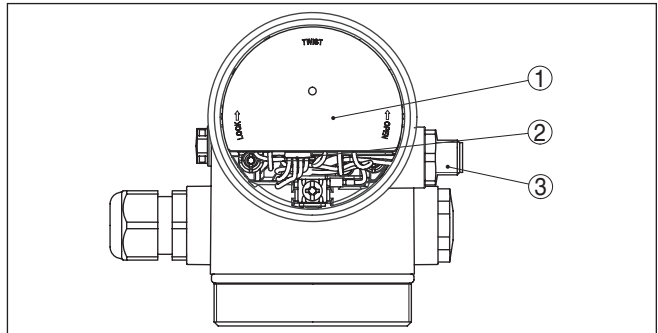
Рис. 11: Вид отсека электроники с адаптером VEGADIS для подключения выносного устройства индикации и настройки
