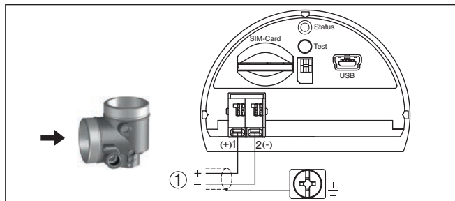
Рис. 14: Отсек подключения встроенного модуля мобильной связи PLICSMOBILE
