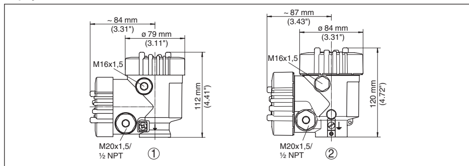
Рис. 38: Размеры корпуса - с установленным модулем индикации и настройки корпус выше на 9 мм (0.35 in)
