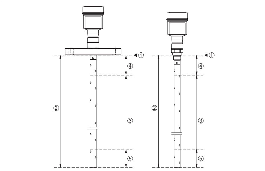
Рис. 33: Диапазоны измерения - VEGAFLEX 81
