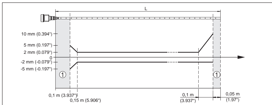
Рис. 35: Погрешность измерения VEGAFLEX 81 в коаксиальном исполнении (среда - масло)
