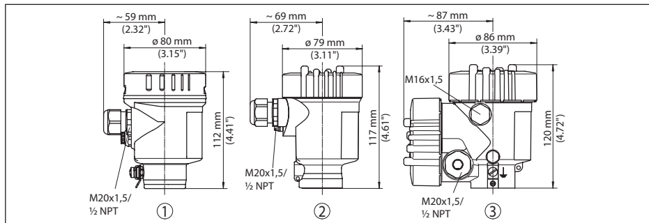
Рис. 46: Корпуса в исполнении IP 66/IP 68 (0,2 bar) - с установленным модулем индикации и настройки корпус выше на 9 мм/0.35 in
