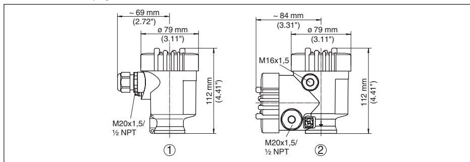
Рис. 43: Корпуса в исполнении со степенью защиты IP 66/IP 67 (с установленным модулем индикации и настройки корпус выше на 9 мм/0.35 in)
