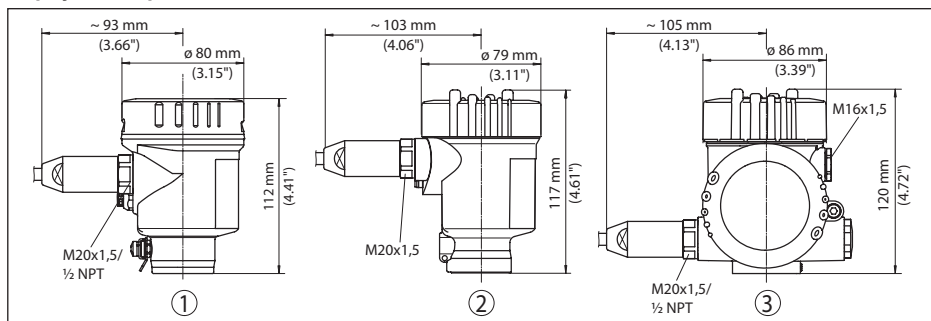
Рис. 47: Корпуса в исполнении IP 66/IP 68 (1 bar) - с установленным модулем индикации и настройки корпус выше на 9 мм/0.35 in
