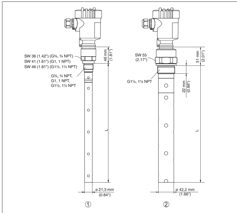
Рис. 48: VEGAFLEX 81, резьбовое исполнение
