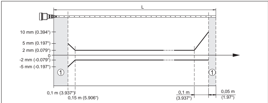
Рис. 40: Погрешность измерения VEGAFLEX 81 в коаксиальном исполнении (среда - масло)
