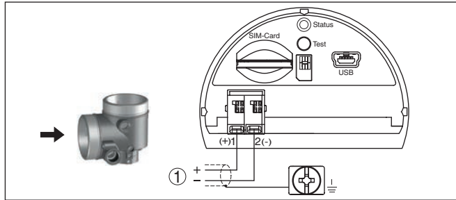
Рис. 19: Отсек подключения встроенного модуля мобильной связи PLICSMOBILE
