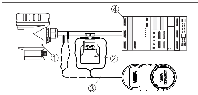
Рис. 25: Подключение ПК к сигнальному кабелю через HART
