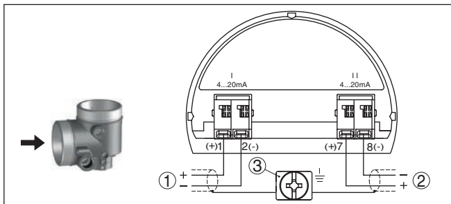
Рис. 18: Отсек подключения в двухкамерном корпусе, дополнительная электроника "Дополнительный токовый выход"
