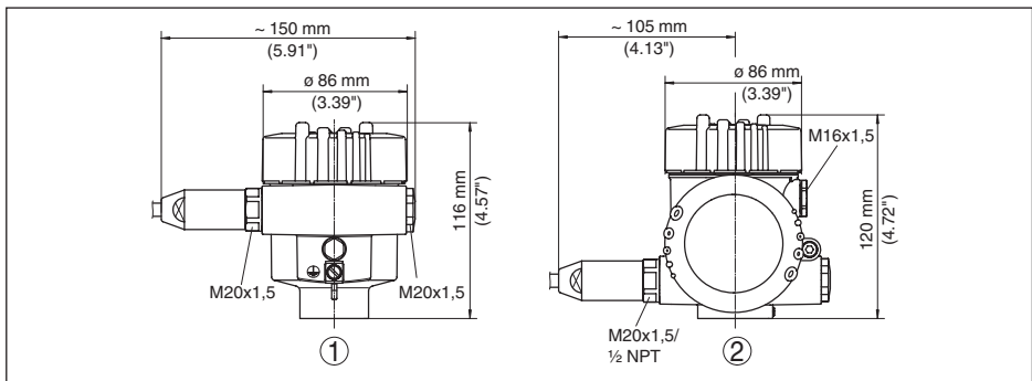
Рис. 45: Корпуса в исполнении IP 66/IP 68 (1 bar) - с установленным модулем индикации и настройки корпус выше на 9 mm/0.35 in
