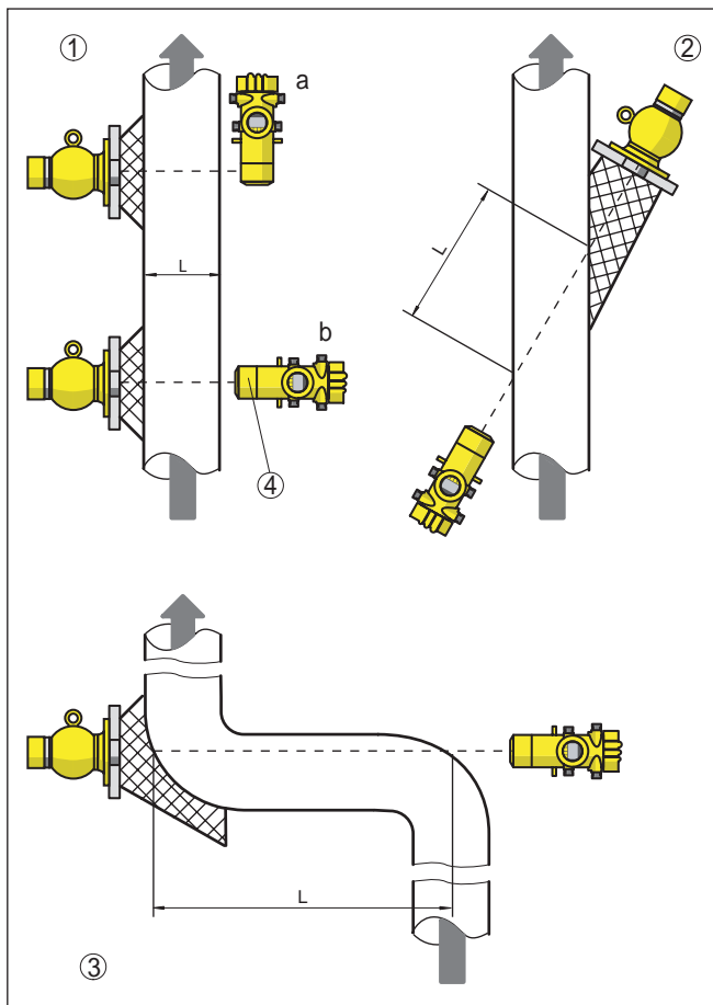
Рис. 5: Варианты монтажа для измерения плотности или концентрации
