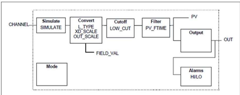
Рис. 24: Схема функционального блока Analog Input (AI)
