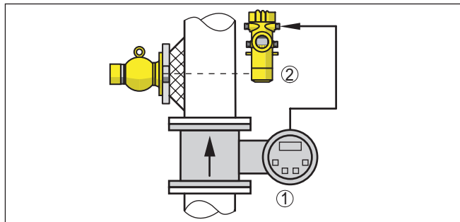
Рис. 6: Измерение массового расхода
