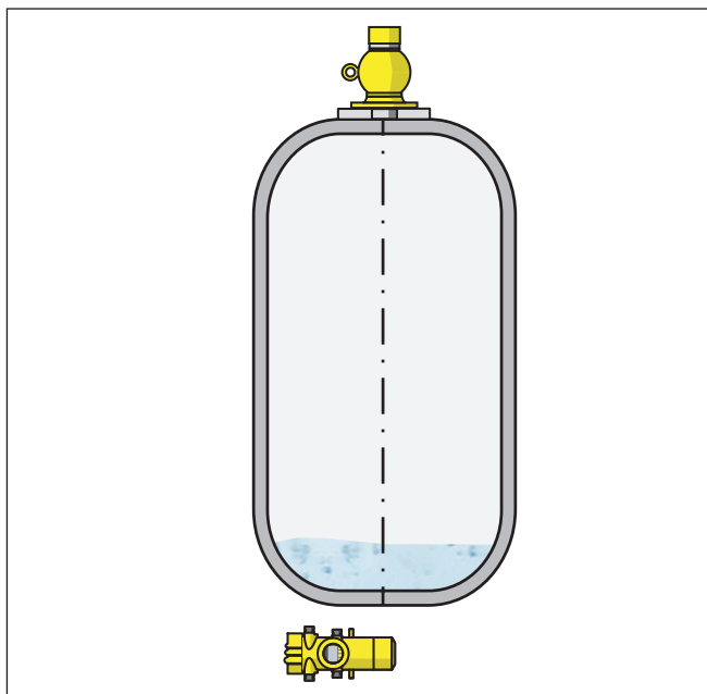
Рис. 8: Измерение уровня - обнаружение остатков в резервуаре-хранилище
