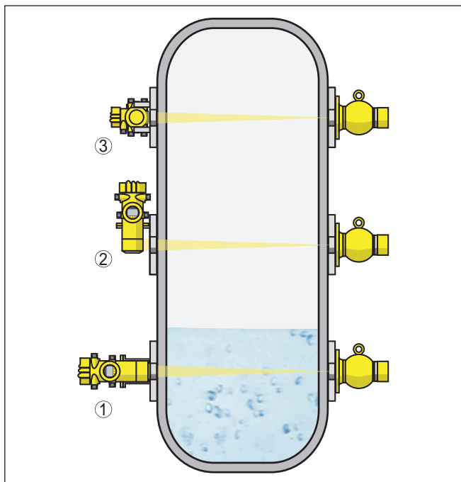
Рис. 7: Монтажная позиция - сигнализация предельного уровня
