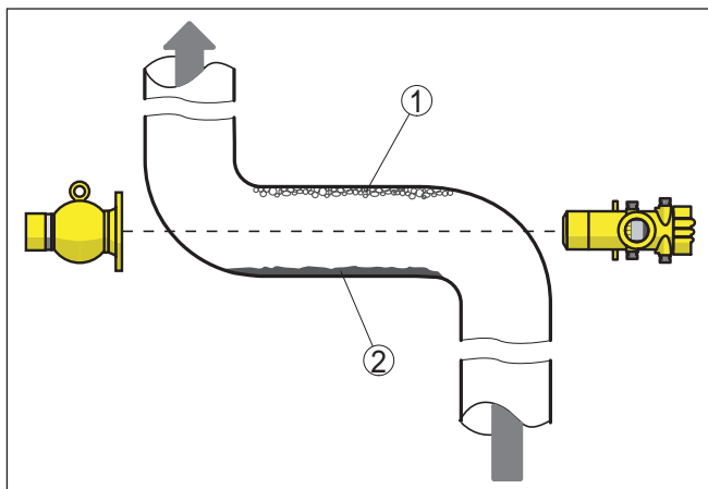
Рис. 4: Монтаж на горизонтальном трубопроводе
