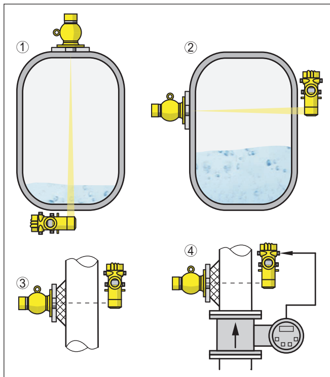
Рис. 2: Возможности применения MINITRAC 31
