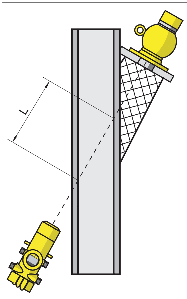
Рис. 20: При косоугольном монтаже применяется длина просвечиваемого отрезка.
