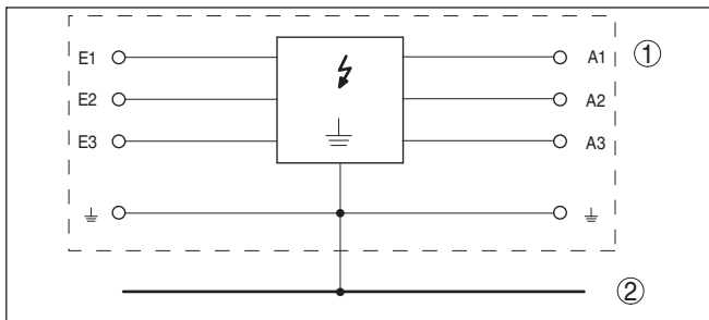
Рис. 7: Принципиальная схема B53-19
