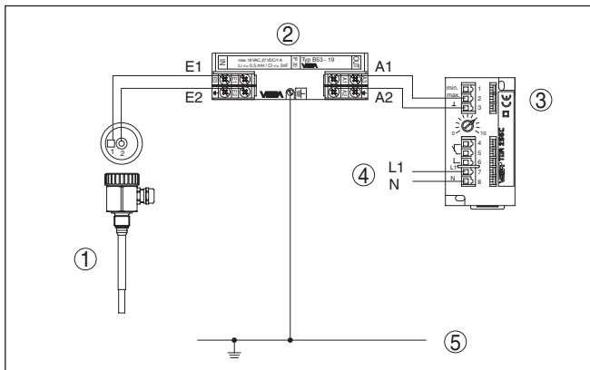
Рис. 8: Схема подключения B53-19 с кондуктивным одностержневым измерительным зондом
