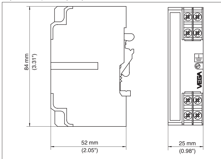
Рис. 10: Размеры В53-19
