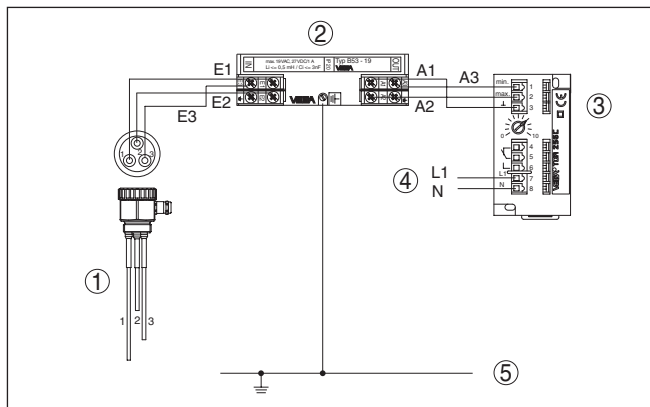
Рис. 9: Схема подключения V53-19 с кондуктивным трехстержневым измерительным зондом
