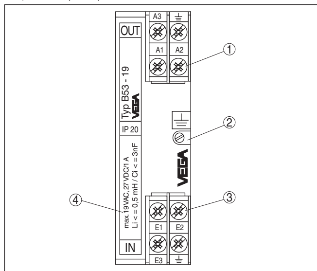
Рис. 1: Конструкция устройства В53-19
