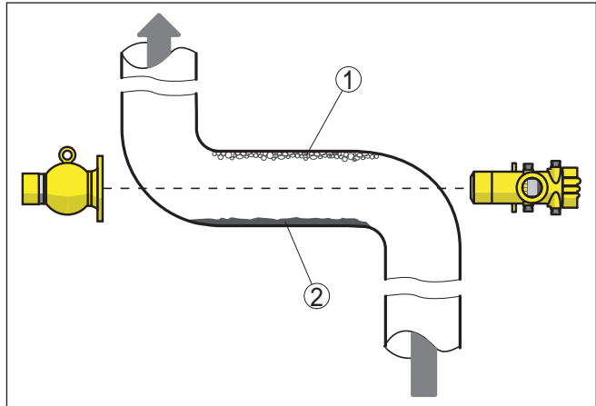
Рис. 4: Монтаж на горизонтальном трубопроводе
