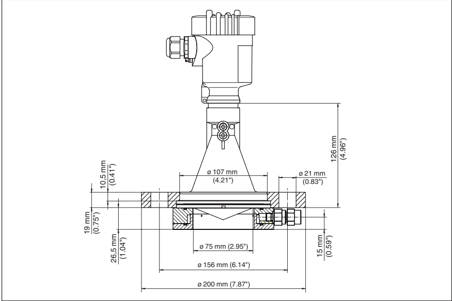
Рис. 69: VEGAPULS 67, исполнение с накидным фланцем и продувочным присоединением, подходит для DN 80 PN 16/ASME 3" 150lbs/JIS80 10K
