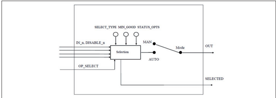
Рис. 60: Схема функционального блока Input Selector
