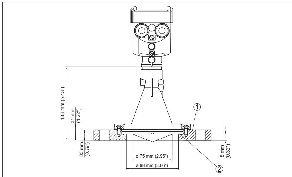
Рис. 70: VEGAPULS 67, адаптерный фланец
