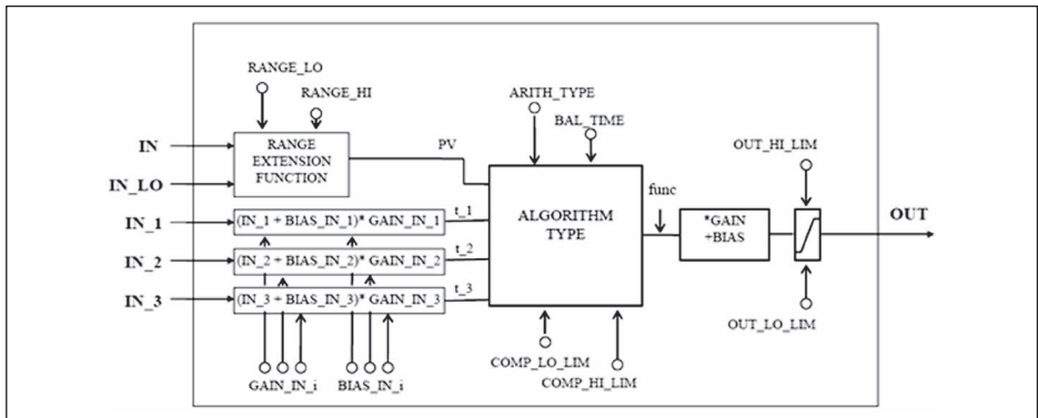
Рис. 61: Схема функционального блока Arithmetic
