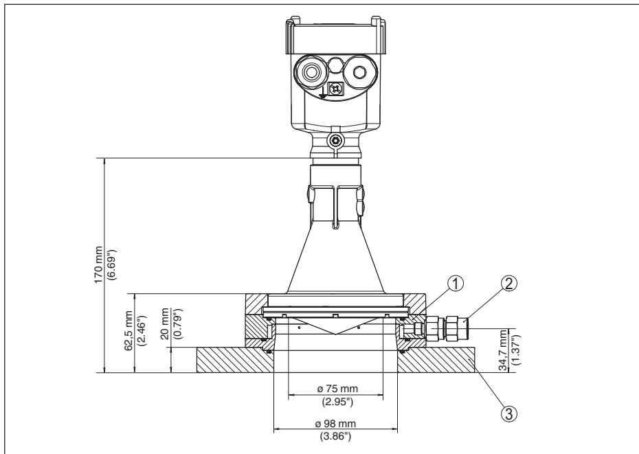
Рис. 71: VEGAPULS 67, адаптерный фланец и продувочное присоединение
