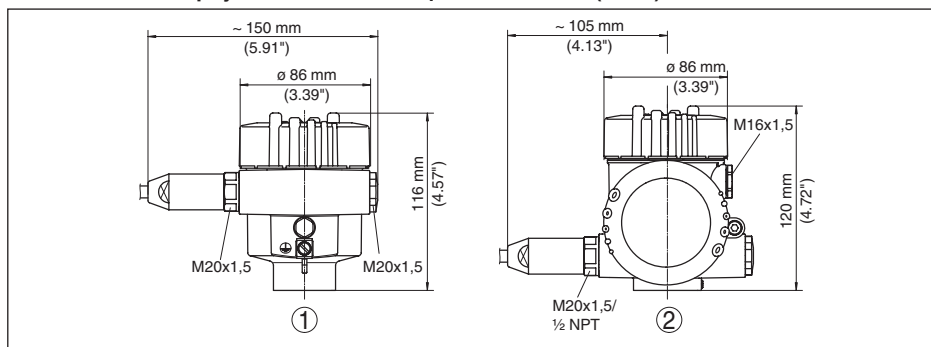
Рис. 52: Корпуса в исполнении IP 66/IP 68 (1 bar) - с установленным модулем индикации и настройки корпус выше на 9 mm/0.35 in
