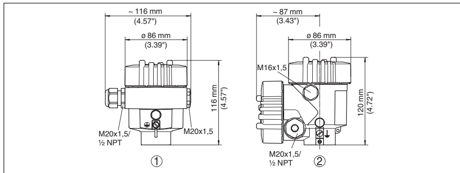
Рис. 51: Корпуса в исполнении IP 66/IP 68 (0,2 bar) - с установленным модулем индикации и настройки корпус выше на 9 mm/0.35 in
