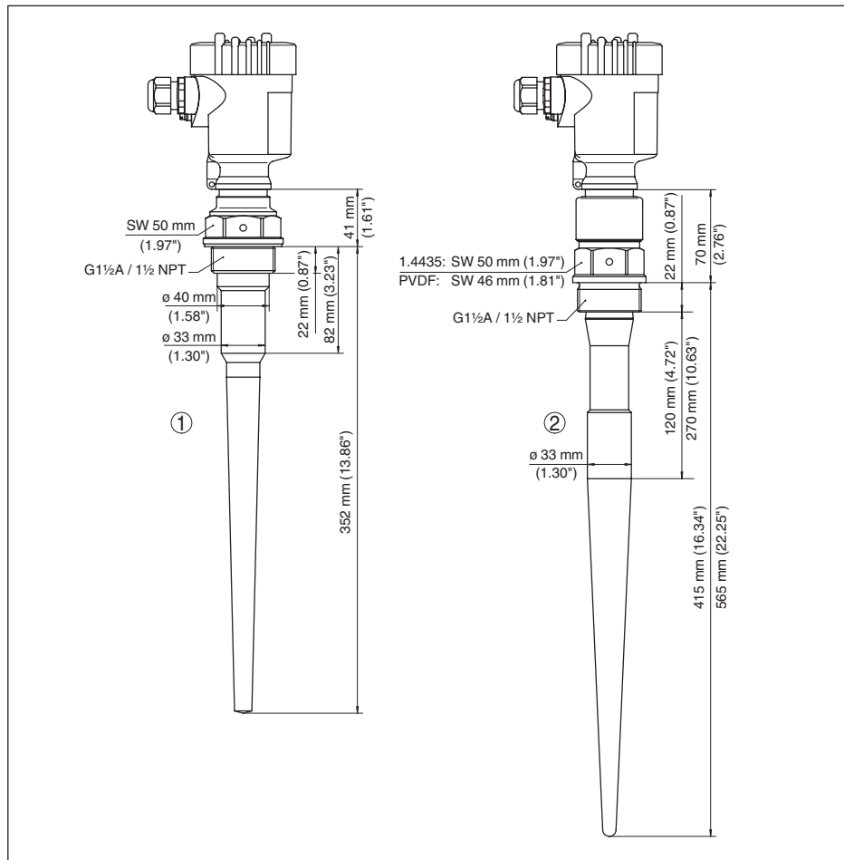
Рис. 53: VEGAPULS 65, резьбовое исполнение
