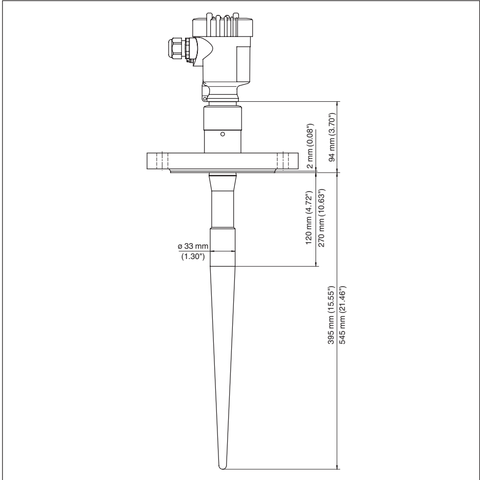
Рис. 54: VEGAPULS 65 во фланцевом исполнении для патрубков высотой 100 мм (неактивная длина 120 мм) или 250 мм (неактивная длина 270 мм)
