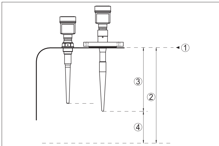
Рис. 39: Данные для входной величины
