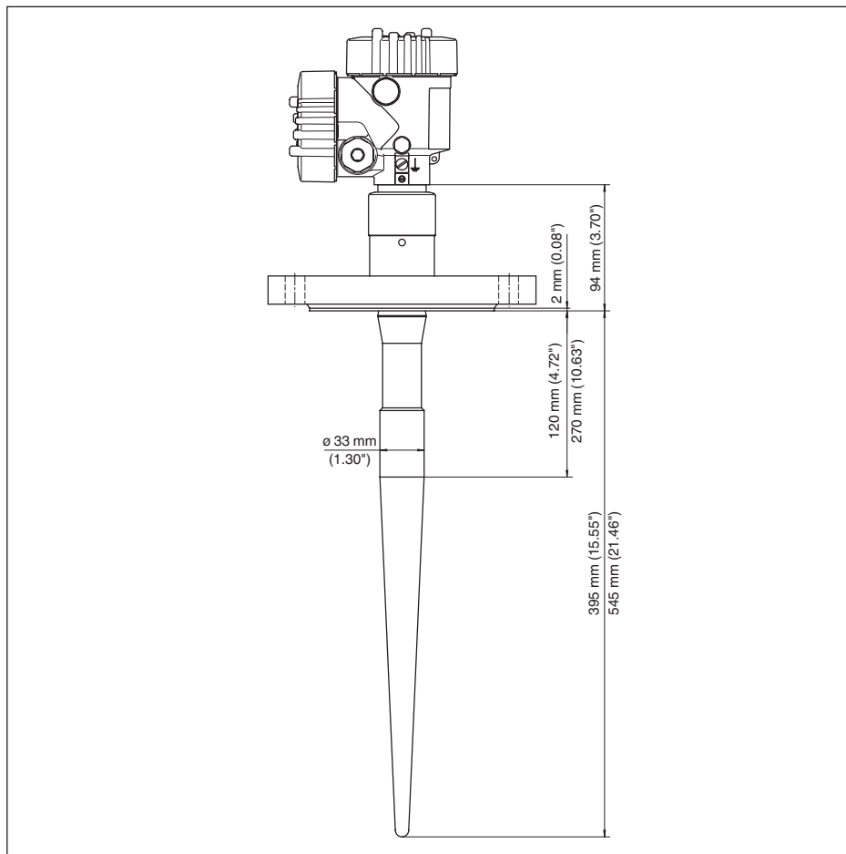
Рис. 43: VEGAPULS 65 во фланцевом исполнении для патрубков высотой 100 мм (неактивная длина 120 мм) или 250 мм (неактивная длина 270 мм)
