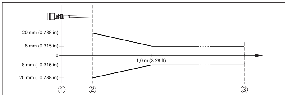
Рис. 40: Погрешность измерения при эталонных условиях
