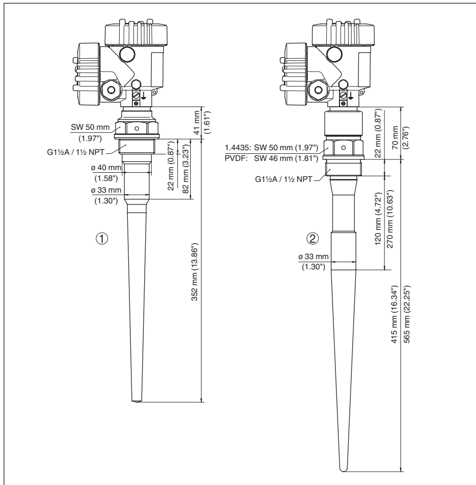
Рис. 42: VEGAPULS 65, резьбовое исполнение
