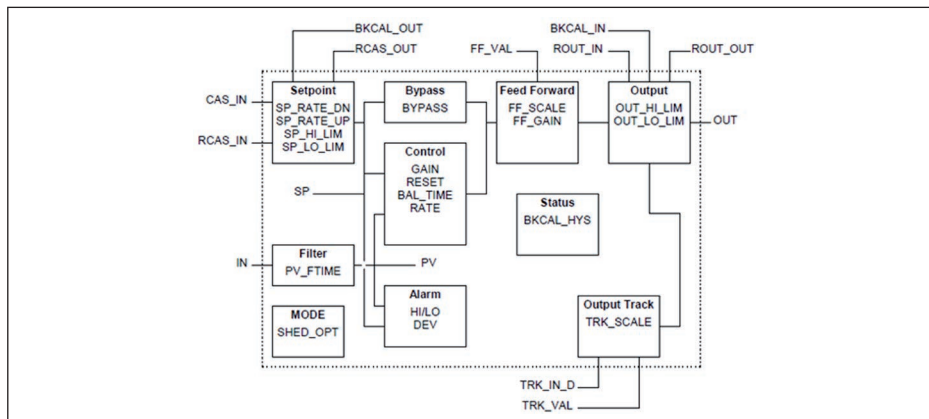
Рис. 61: Схема функционального блока PID Control
