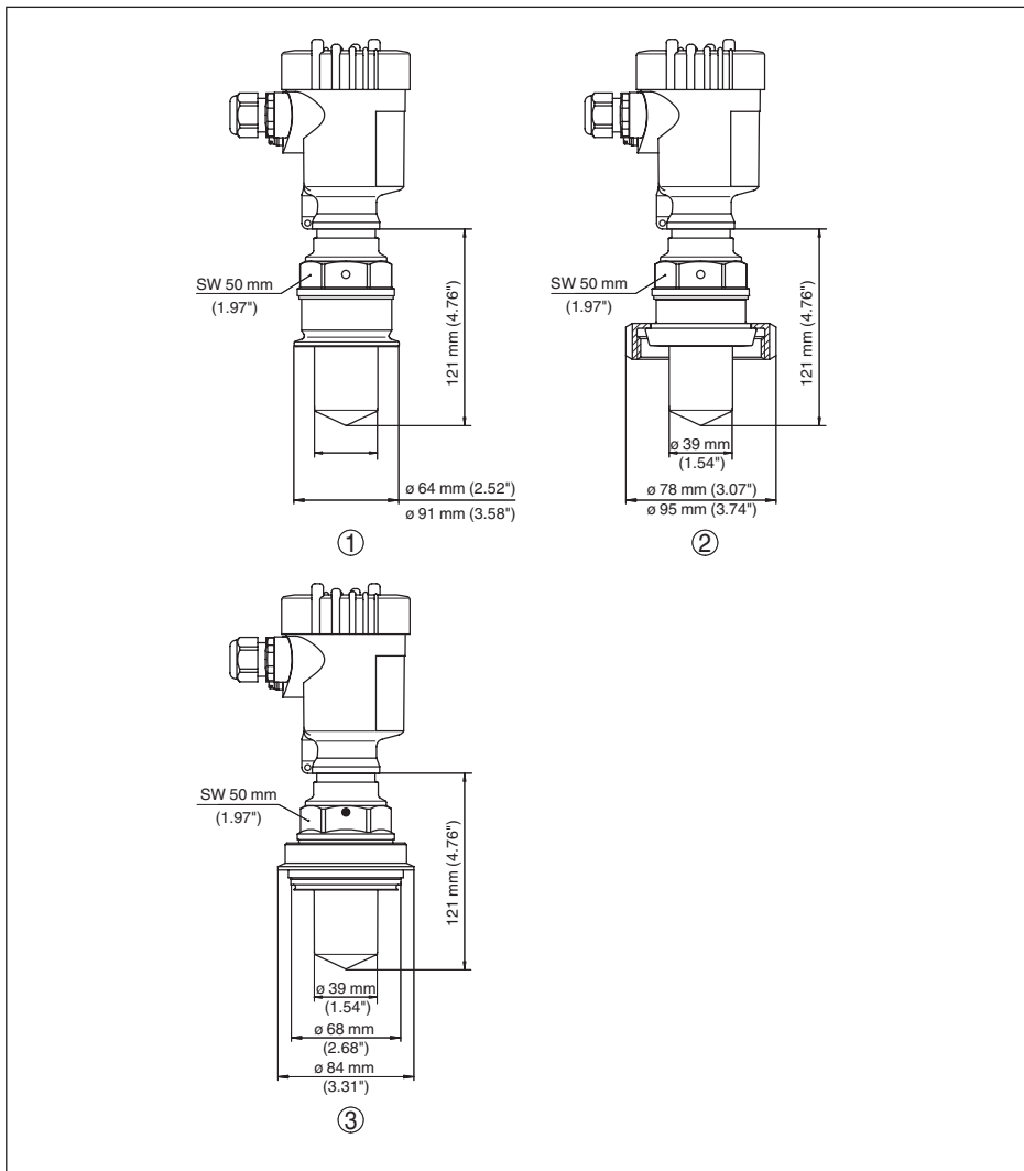
Рис. 73: VEGAPULS 61, гигиеническое присоединение
