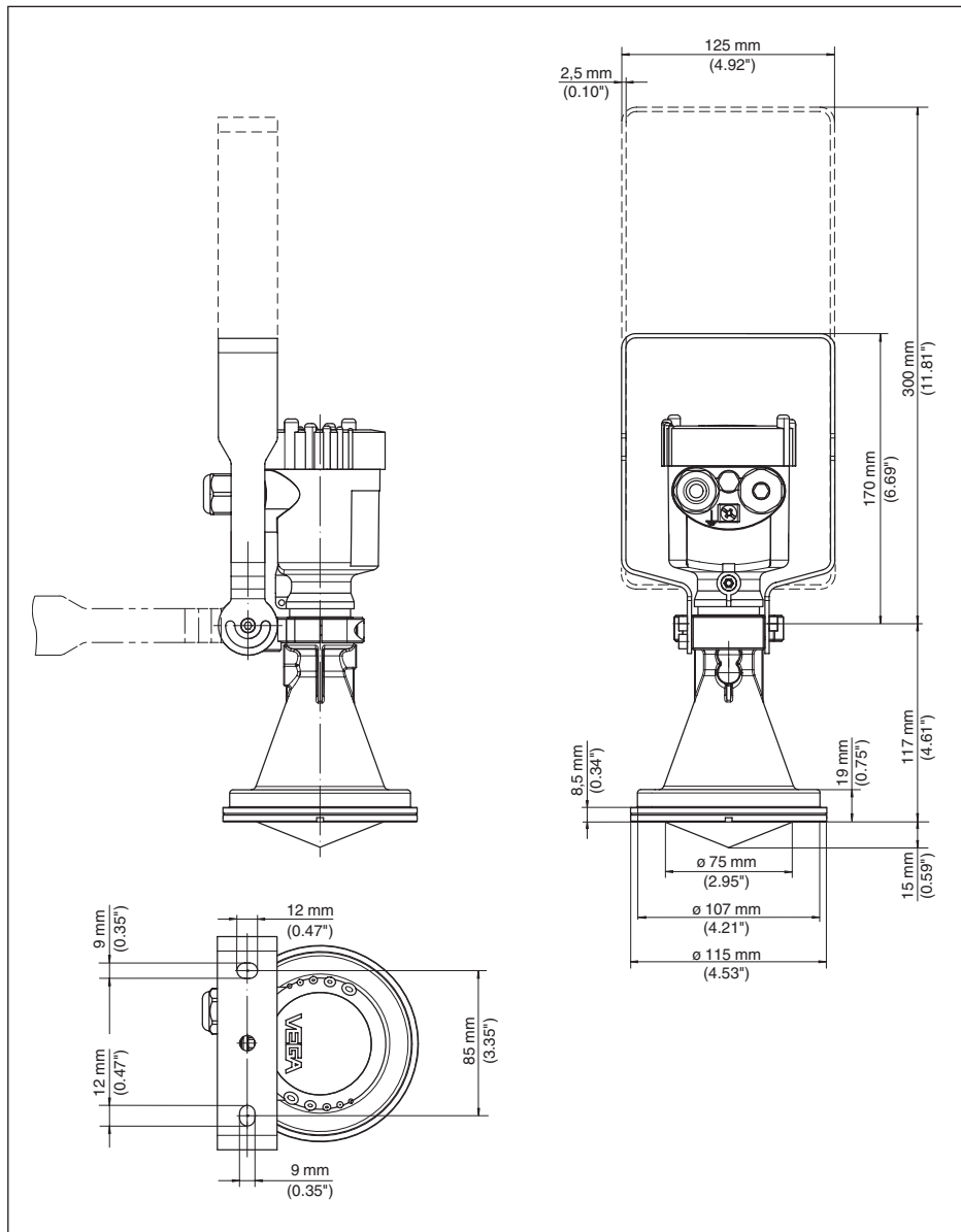
Рис. 75: VEGAPULS 61, монтажная скоба длиной 170 или 300 мм
