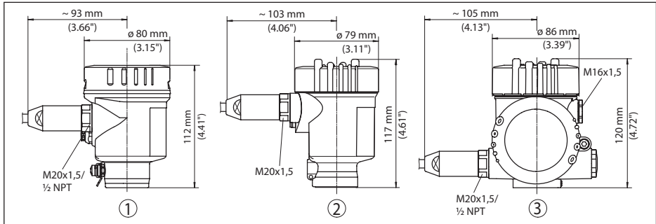
Рис. 71: Корпуса в исполнении IP 66/IP 68 (1 bar) - с установленным модулем индикации и настройки корпус выше на 9 мм/0.35 in
