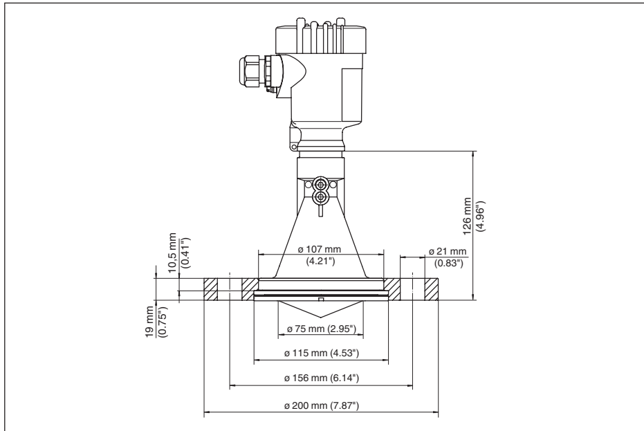
Рис. 77: VEGAPULS 61, накидной фланец для DN 80 PN 16/ASME 3" 150lbs/JIS80 10K
