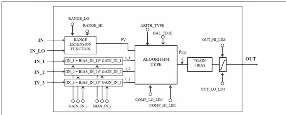
Рис. 66: Схема функционального блока Arithmetic
