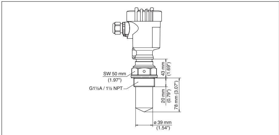
Рис. 72: VEGAPULS 61, резьбовое исполнение G1 1/2 и 1 1/2 NPT
