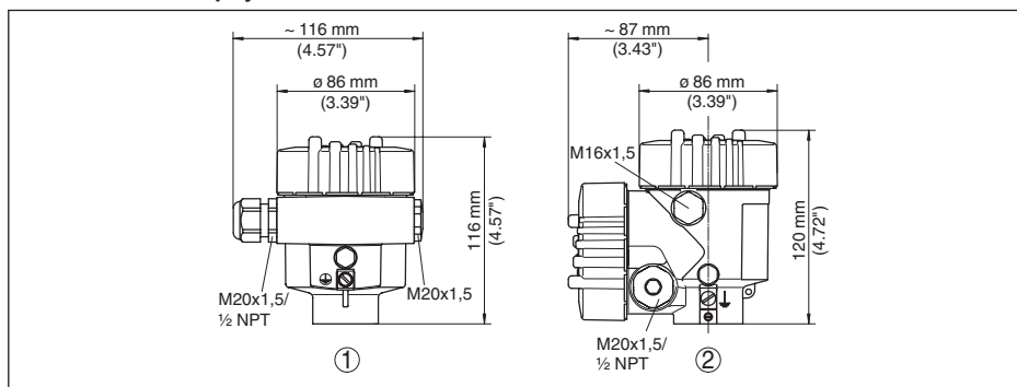
Рис. 68: Корпуса в исполнении IP 66/IP 68 (0,2 bar) - с установленным модулем индикации и настройки корпус выше на 9 мм/0.35 in
