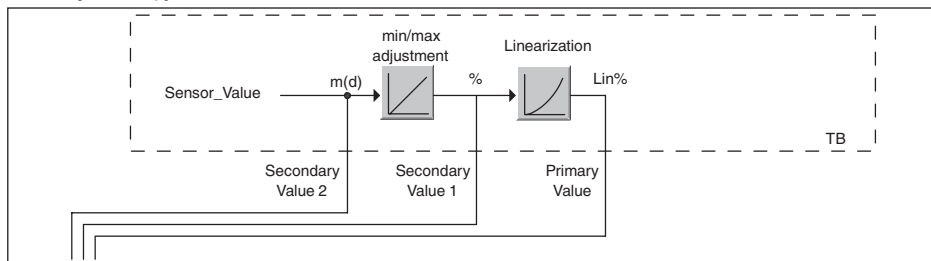
Рис. 58: Схематическое представление блока преобразователя (TB)
