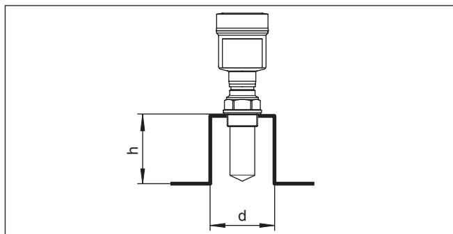
Рис. 10: Ориентировочные размеры патрубков
