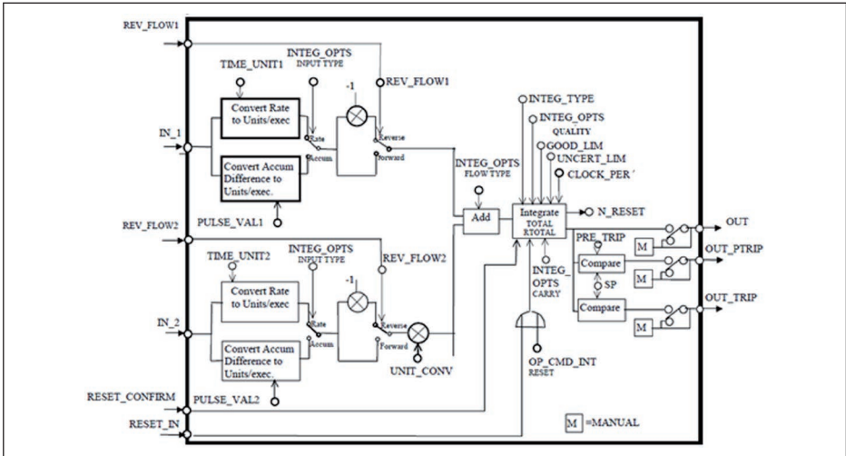
Рис. 64: Схема функционального блока Integrator
