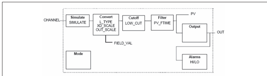
Рис. 59: Схема функционального блока Analog Input (AI)
