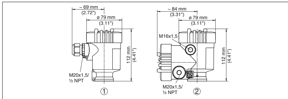
Рис. 67: Корпуса в исполнении со степенью защиты IP 66/IP 67 (с установленным модулем индикации и настройки корпус выше на 9 мм/0.35 in)
