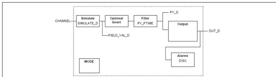
Рис. 60: Схема функционального блока Discret Input (DI)
