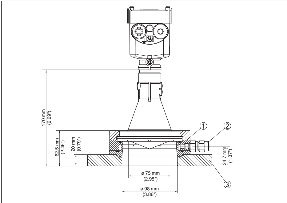
Рис. 80: VEGAPULS 61, адаптерный фланец и продувочное присоединение
