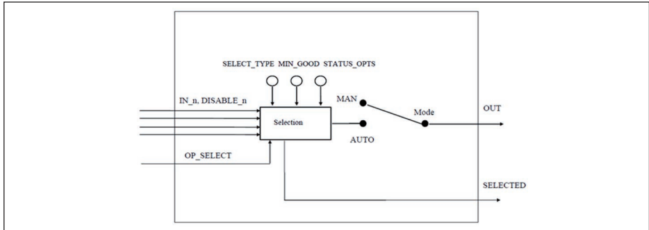
Рис. 65: Схема функционального блока Input Selector
