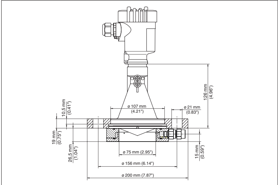
Рис. 78: VEGAPULS 61, исполнение с накидным фланцем и продувочным присоединением, подходит для DN 80 PN 16/ASME 3" 150lbs/JIS80 10K
