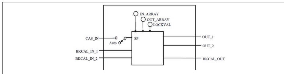
Рис. 62: Схема функционального блока Output Splitter
