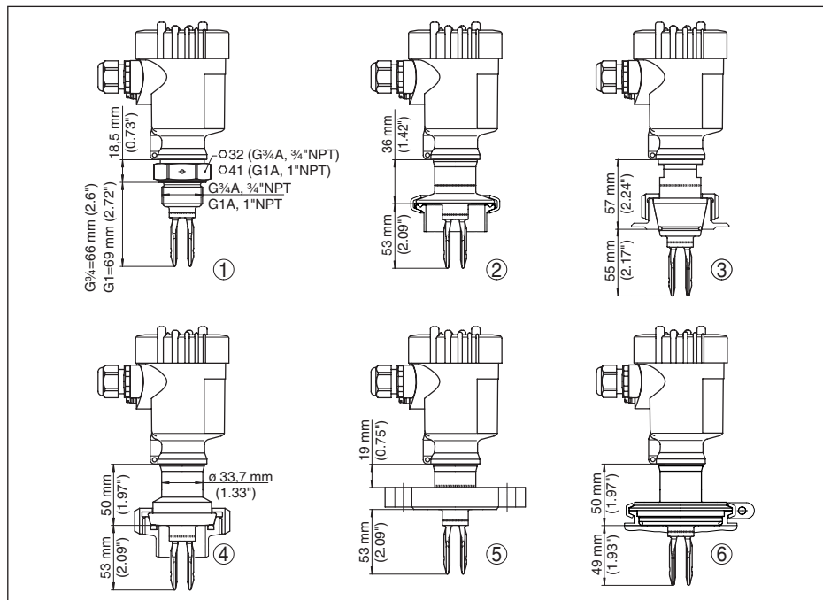
Рис. 35: VEGASWING 61
