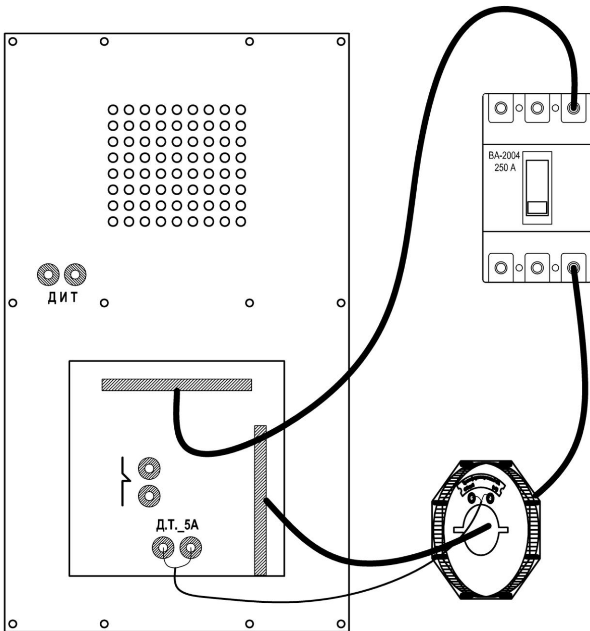
Схема функциональная поверки трехполюсных автоматических выключателей (вариант №1)
