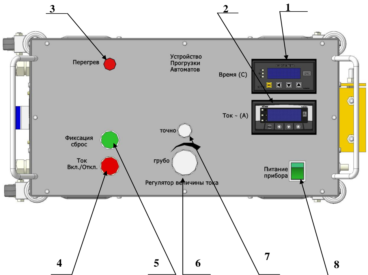
Рис№1. Лицевая сторона прибора УПА–10М
