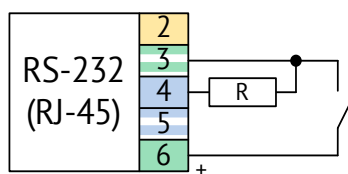
Рисунок 3.5. Схема подключения дополнительного дискретного входа.
