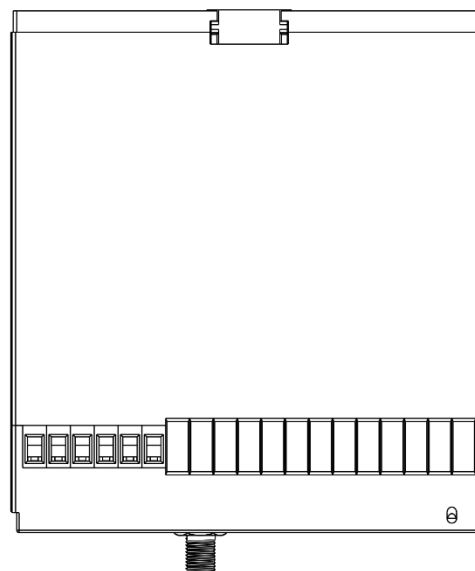
Рисунок 1.6. Габаритные размеры ЭНКМ-3-Х-Х-XXX
