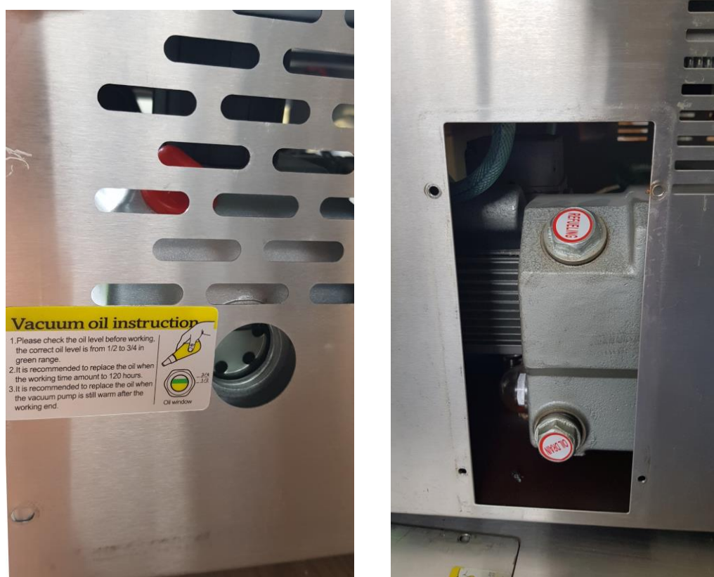
Рис.4.12 - Смотровое окошко для оценки уровня масла
