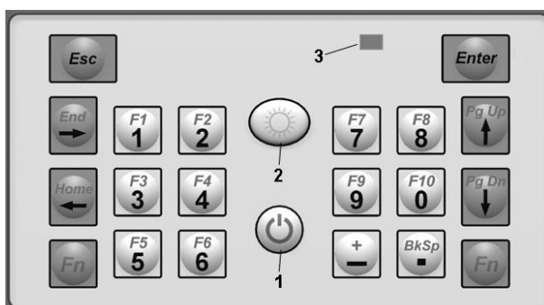
Рис.2в. Клавиатура управления прибором ЛИДЕР-KTM-250.
