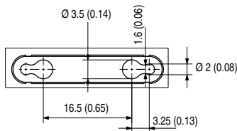
1492-MWT5X23
