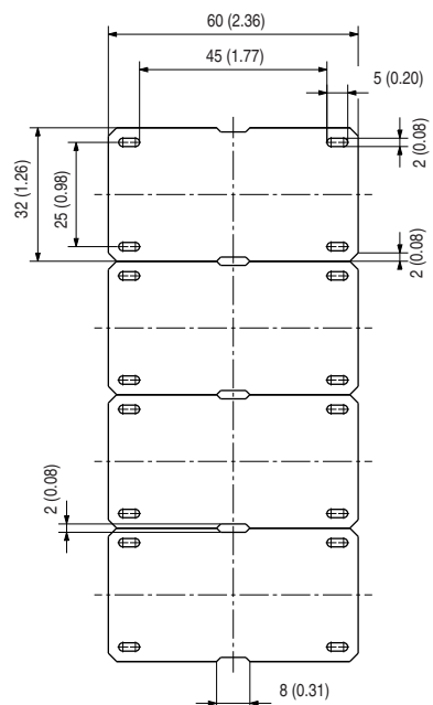
1492-MWCT30X60
