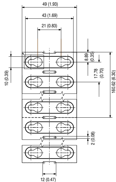
1492-MWT10X23
