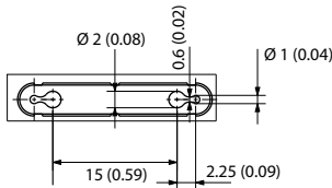
1492-MWT4X23
