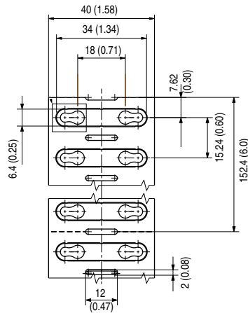
1492-MWT6X23
