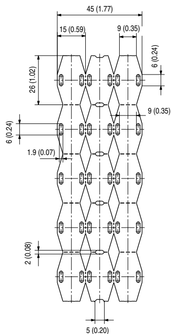
1492-MWCT9X24
