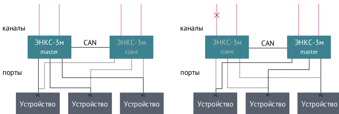
Рисунок 5.2. Проверка каналов.
