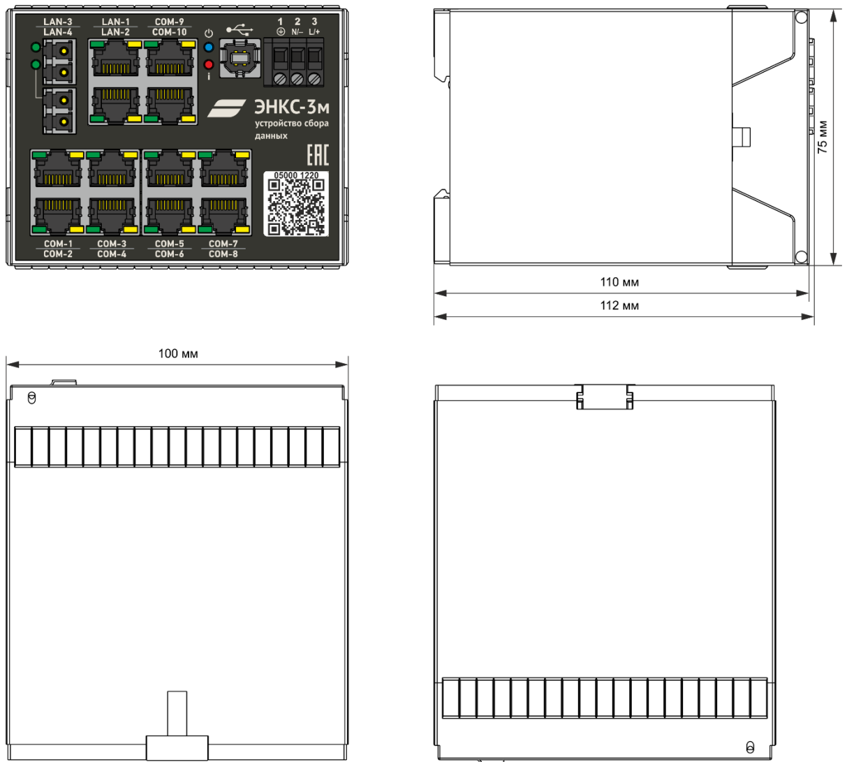
Рисунок 1.7. Габаритные размеры модификации ЭНКС-3м.648-Х-4(5)
