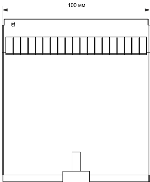
Рисунок 1.6. Габаритные размеры модификации ЭНКС-3м.648-Х-3
