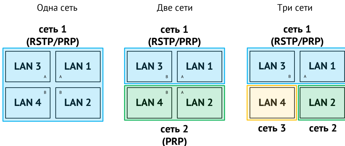
Рисунок 2.3. Режимы работы портов Ethernet в ЭНКС-3м.648...-3(4/5)
