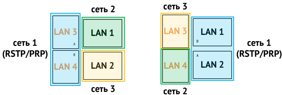
Рисунок 2.4. Варианты работы портов Ethernet в ЭНКС-3м.648...-4/5 для 3 сетей
