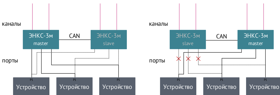
Рисунок 5.3. Проверка портов.
