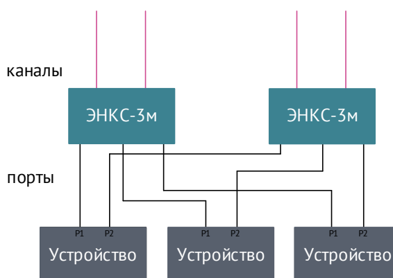
Рисунок 5.1. Дублирование ЭНКС-3м.
