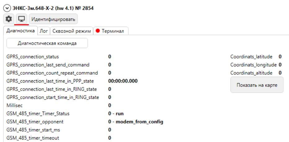
Рисунок 2.6. Интерфейс окна диагностики модема.
