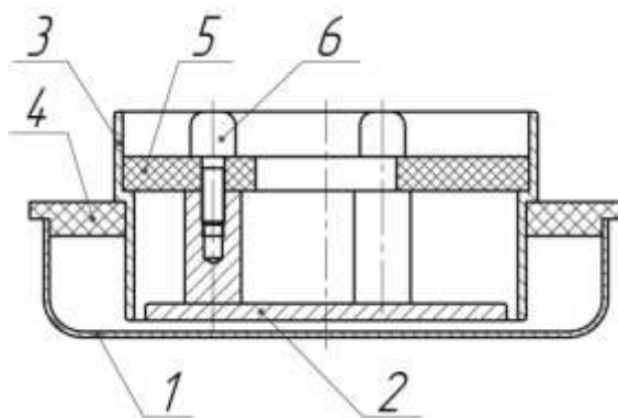
Рисунок 5. Ячейка измерительная:
