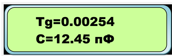
Рисунок 10. Вид экрана модуля индикации «ТАНГЕНС-3М-3-МИ» в режиме измерения тангенса угла диэлектрических потерь и емкости выбранной ячейки.
