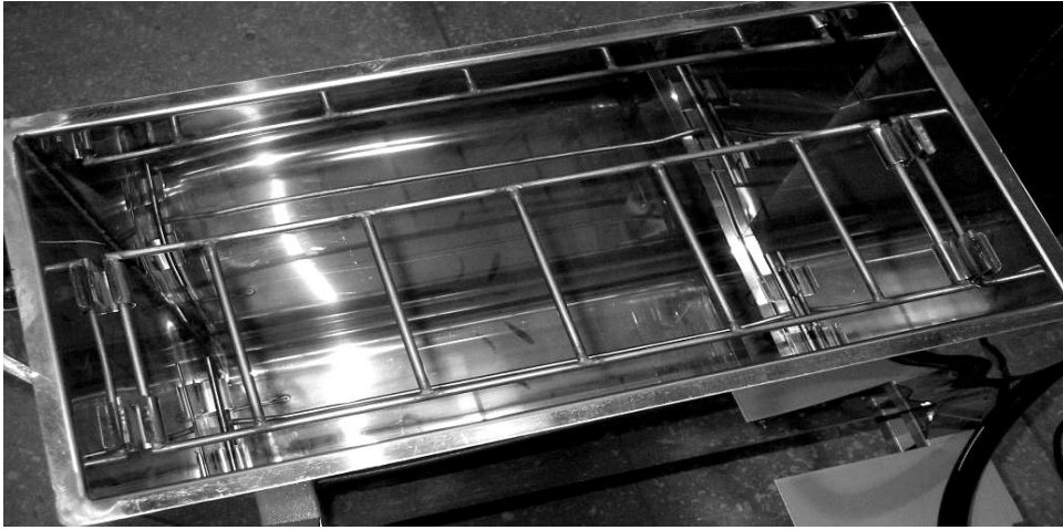
Рис. 8.10. Размещение решетки в ванной.
