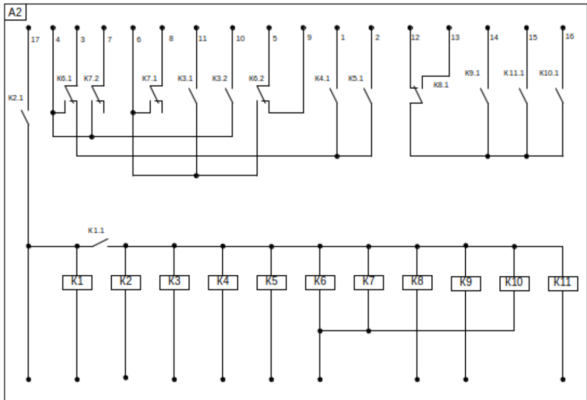
Приложение 3 Стенд высоковольтный стационарный СВС-50 Блок управления. Плата питания А1. Плата коммутации А2. Схема электрическая принципиальная
