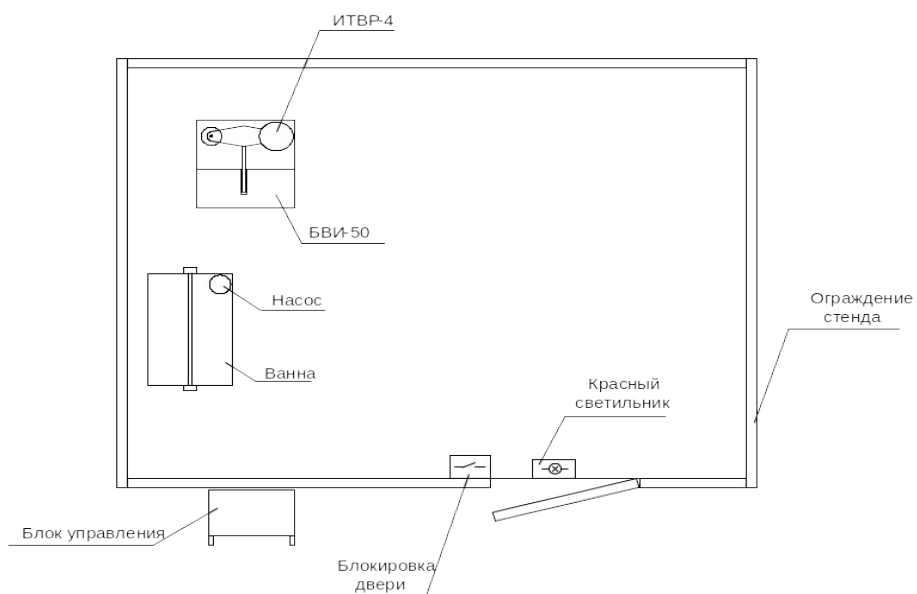
Рис. 4.1 Схема размещения оборудования стенда СВС-50
