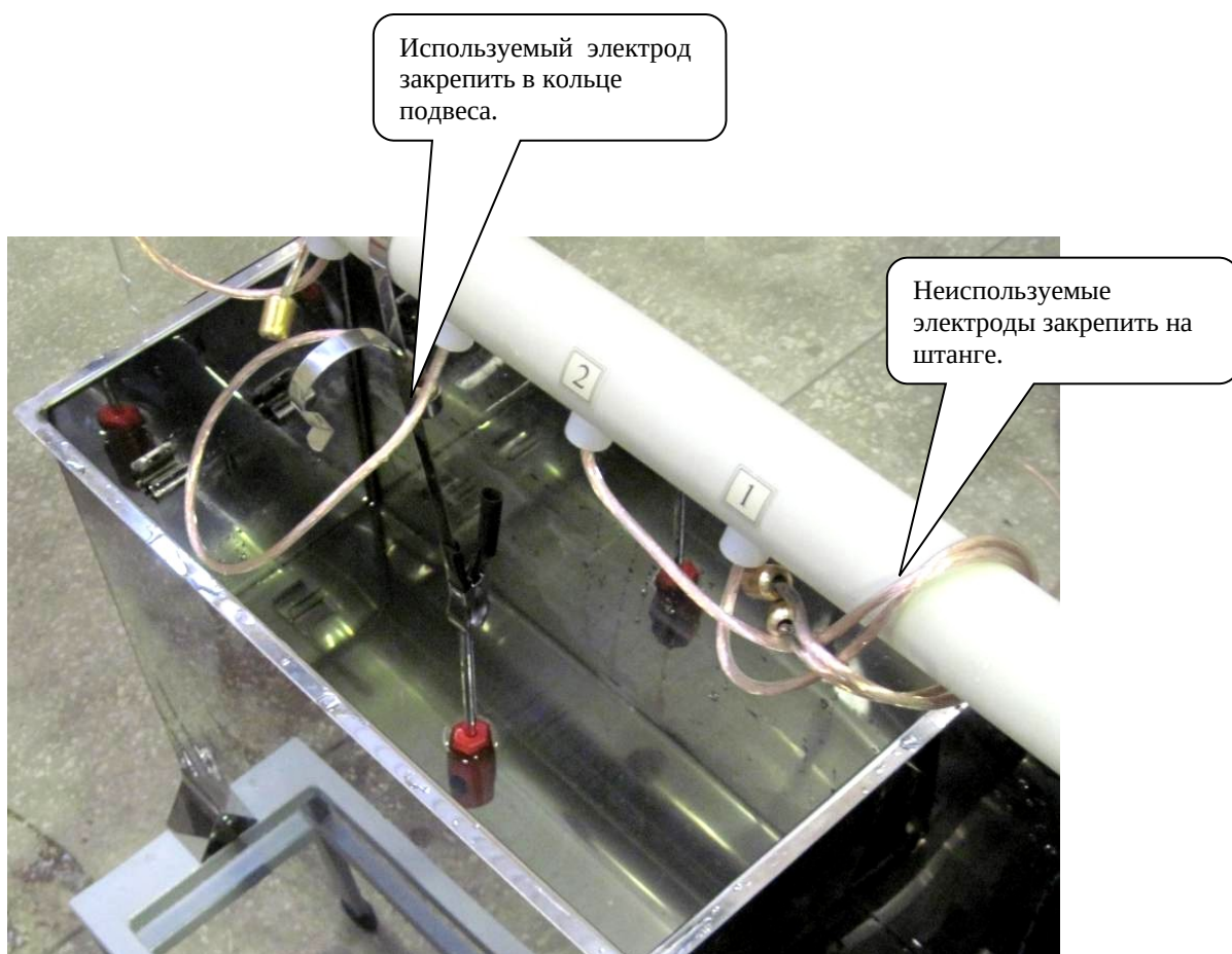
Рис. 4.1 Схема размещения оборудования стенда СВС-50
