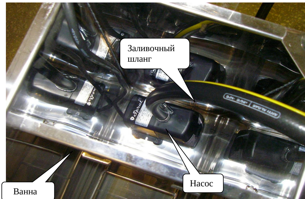
Рис. 7.2.Размещение насоса внутри ванны.
