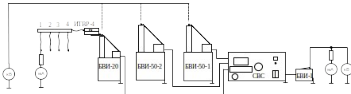
Рисунок 1. Схема определения метрологических характеристик СВС-100.
